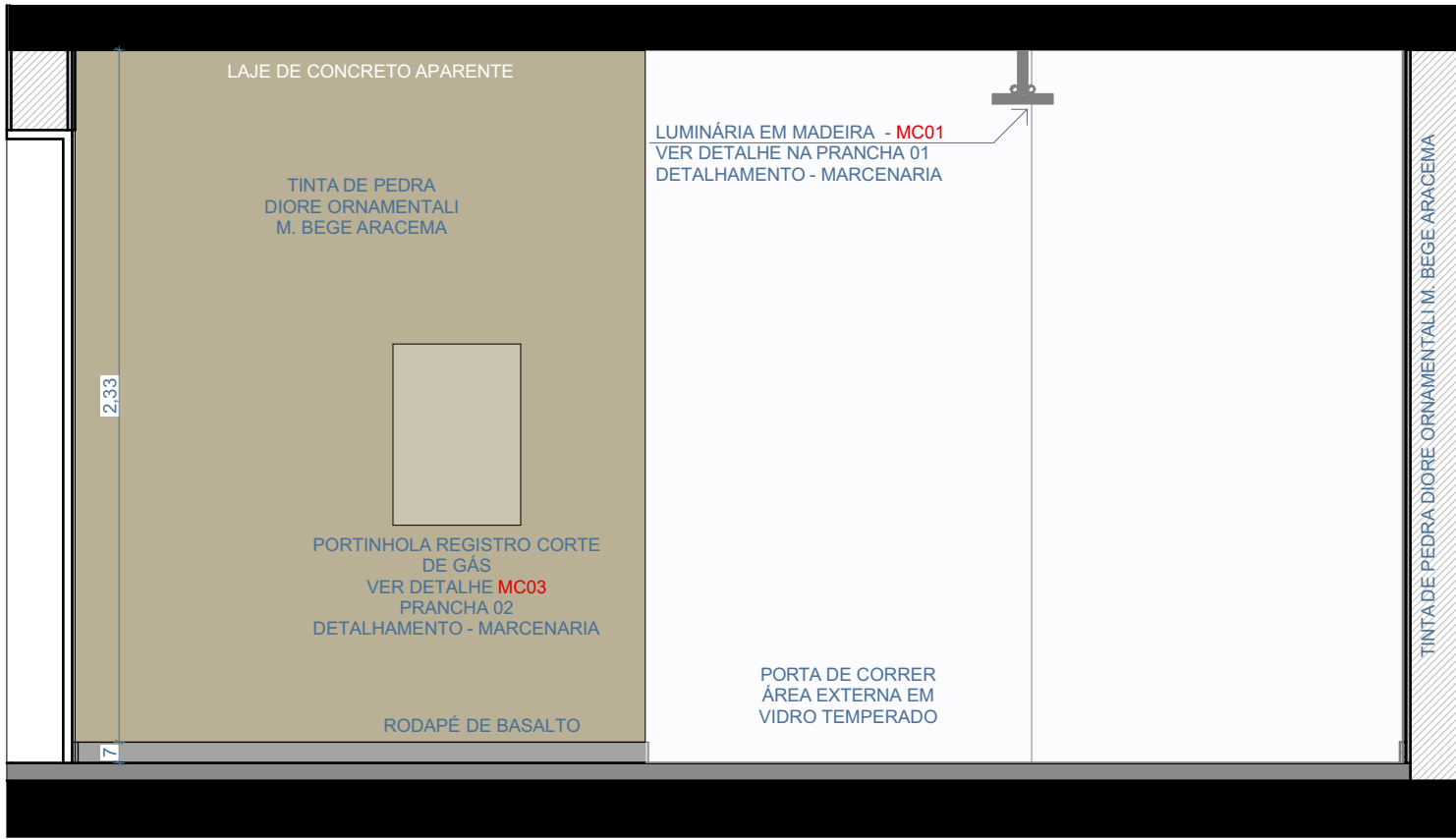
04 ESCALA 1:25
