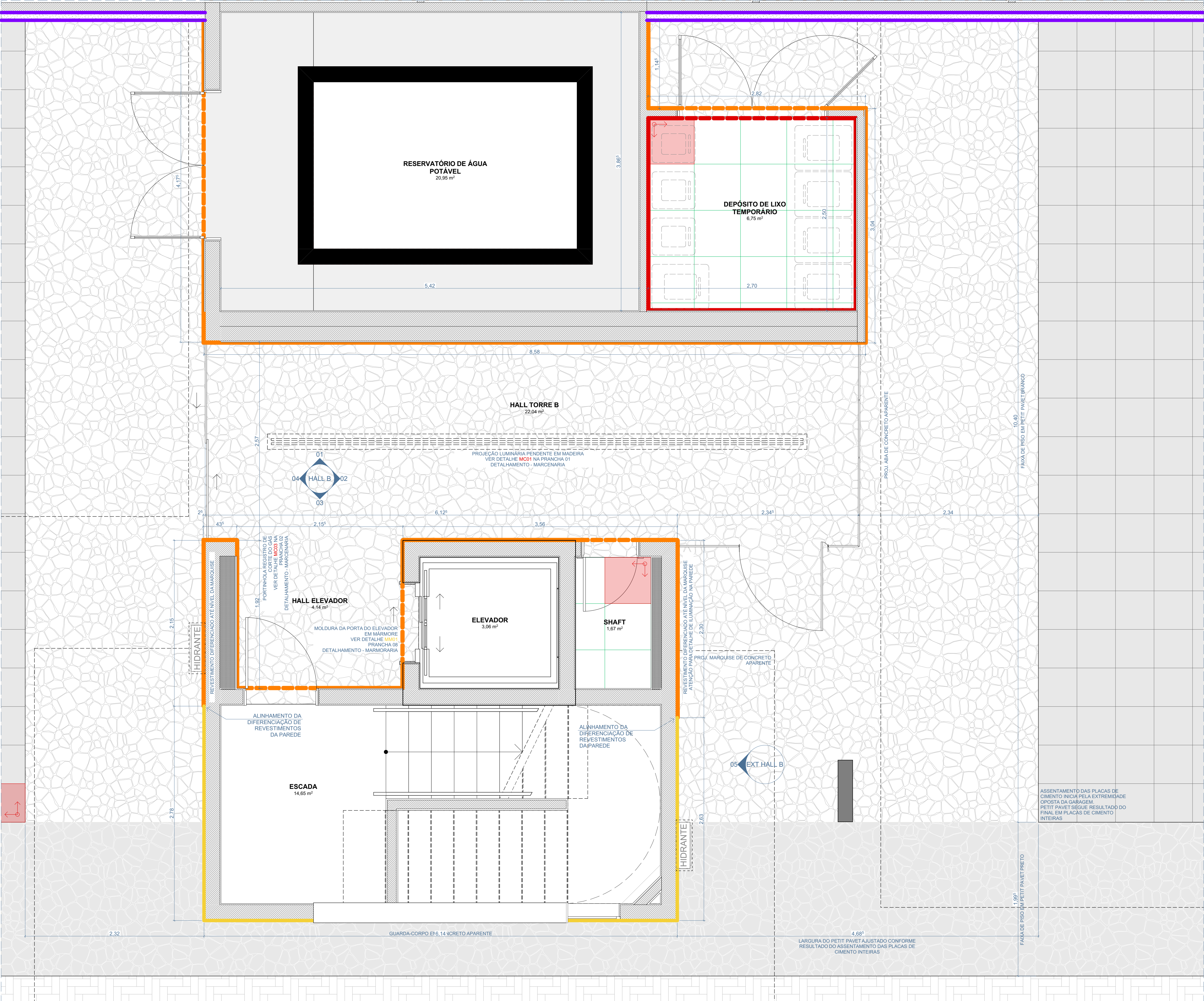
PLANTA BAIXA - HALL B ESCALA 1:25
