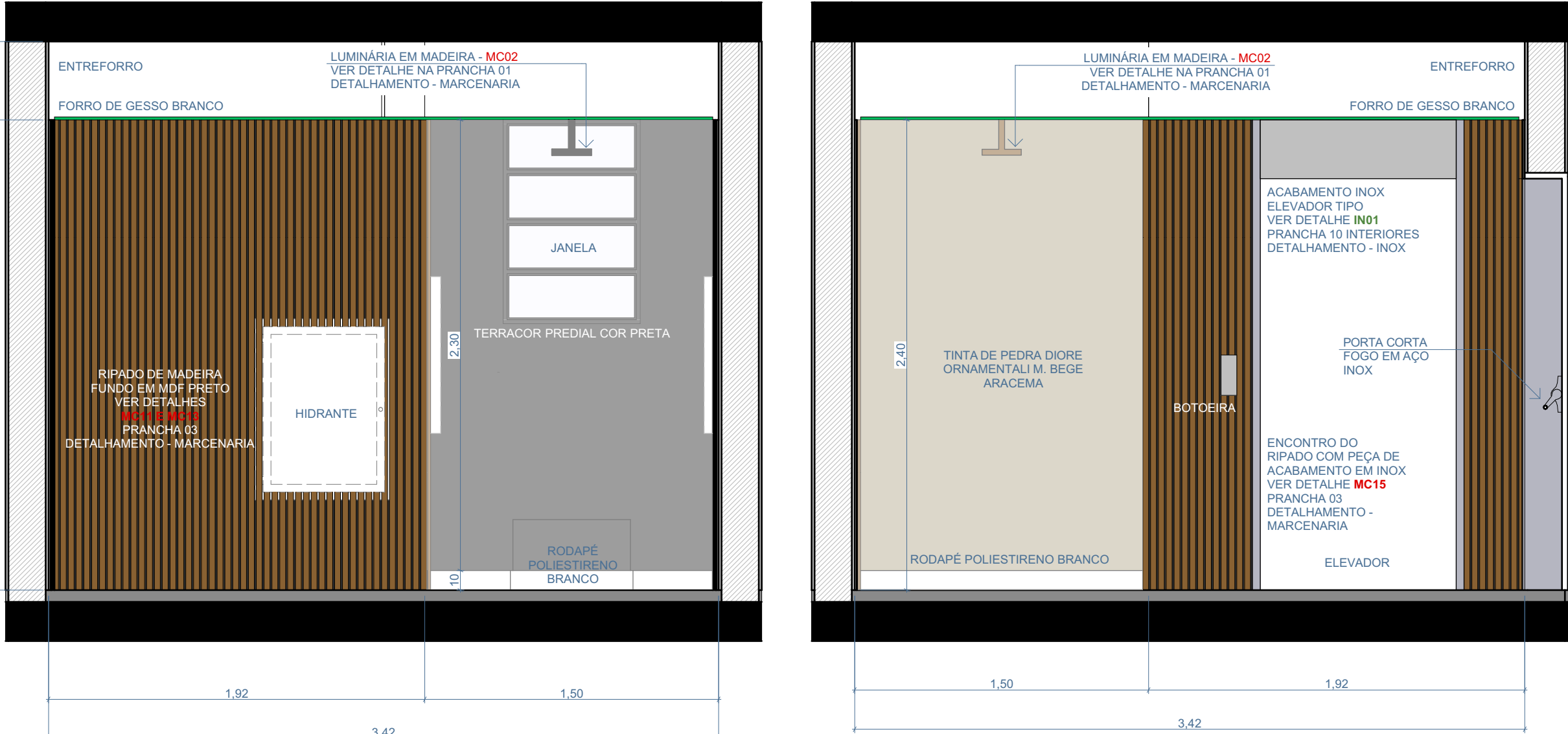
04 B ESCALA 1:25
