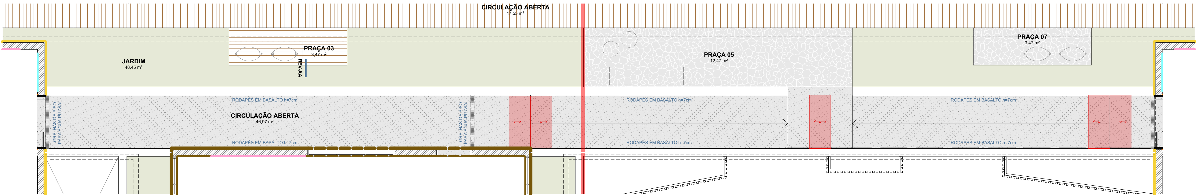
PLANTA BAIXA CIRCULAÇÃO INTERMEDIÁRIA ESCALA 1:50
