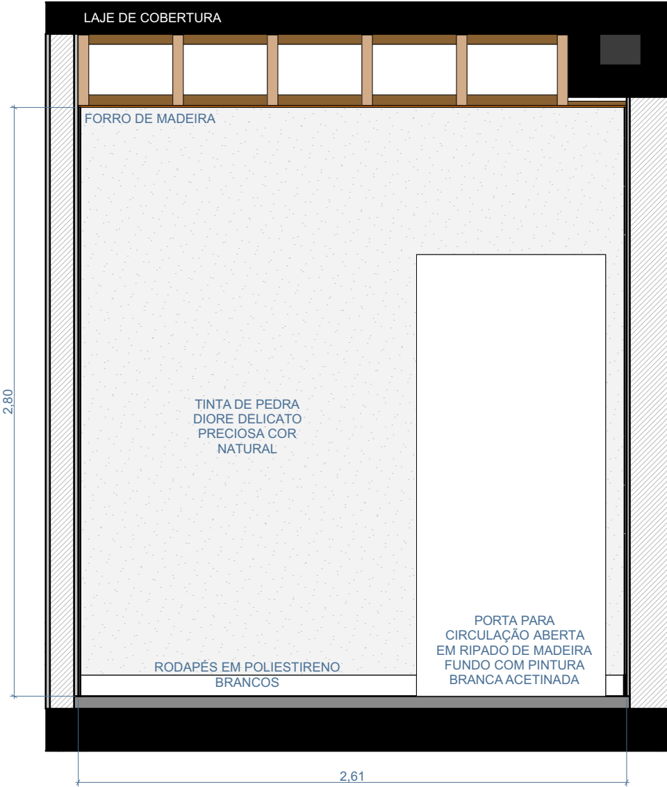
03 ESCALA 1:25
