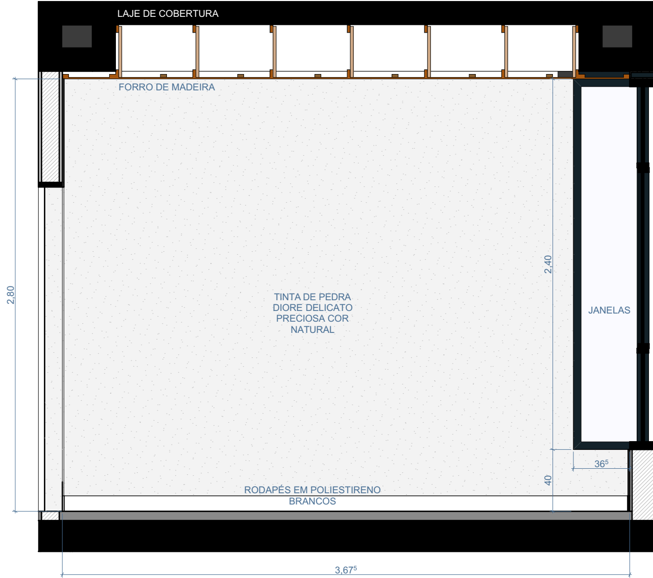
04 ESCALA 1:25
