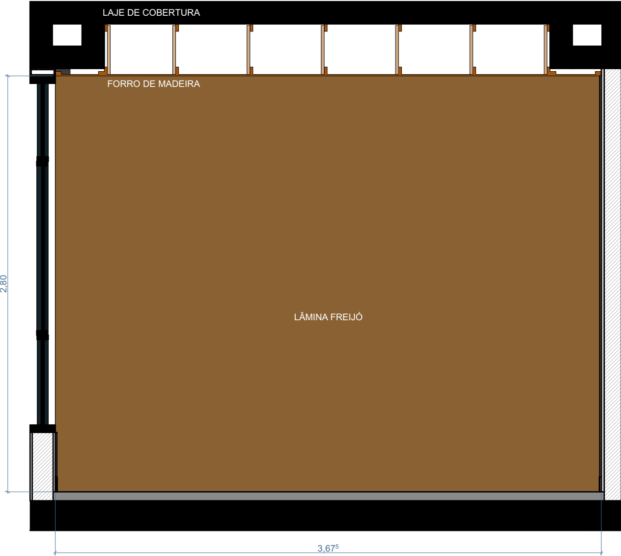
02 ESCALA 1:25
