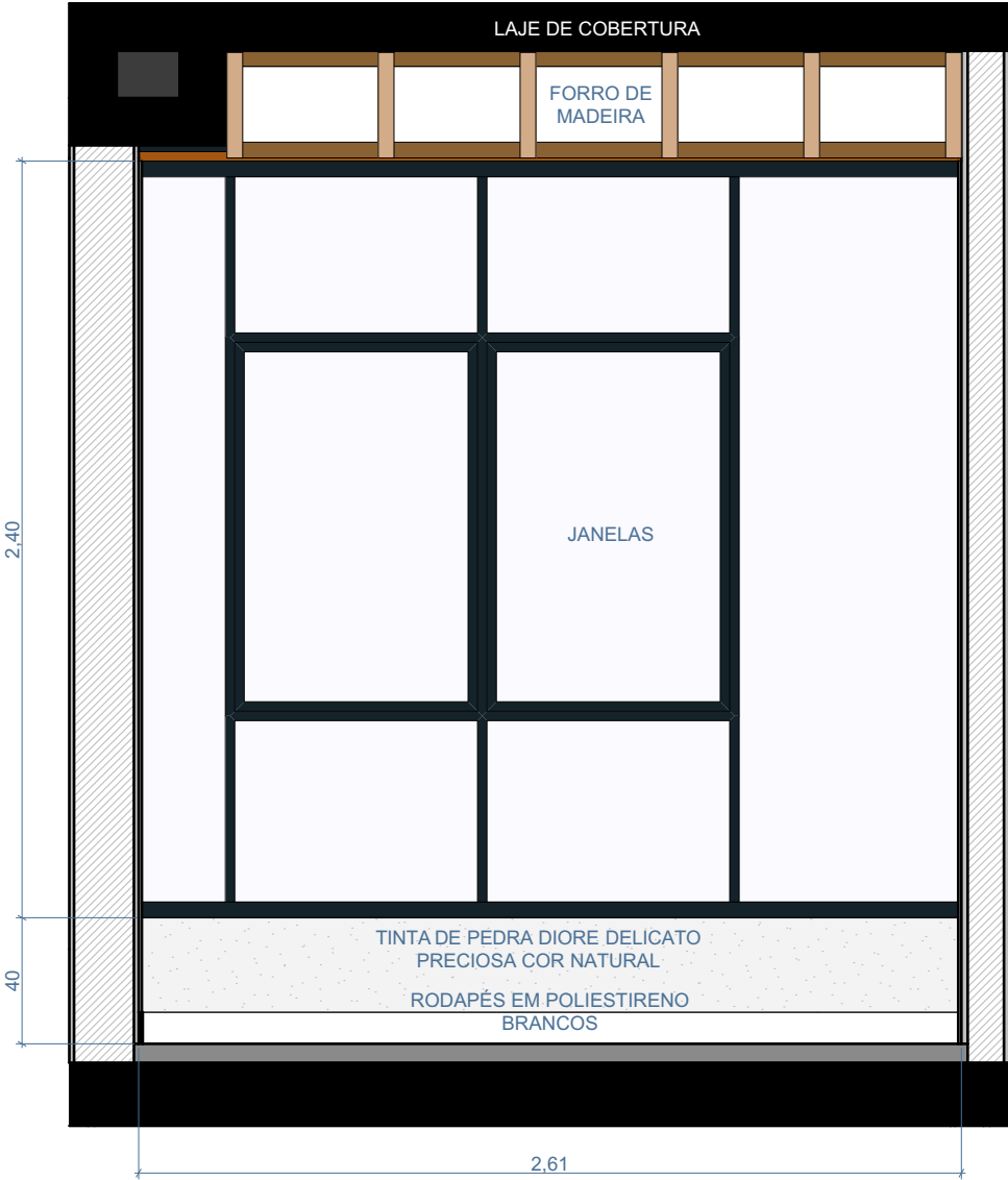
01 ESCALA 1:25
