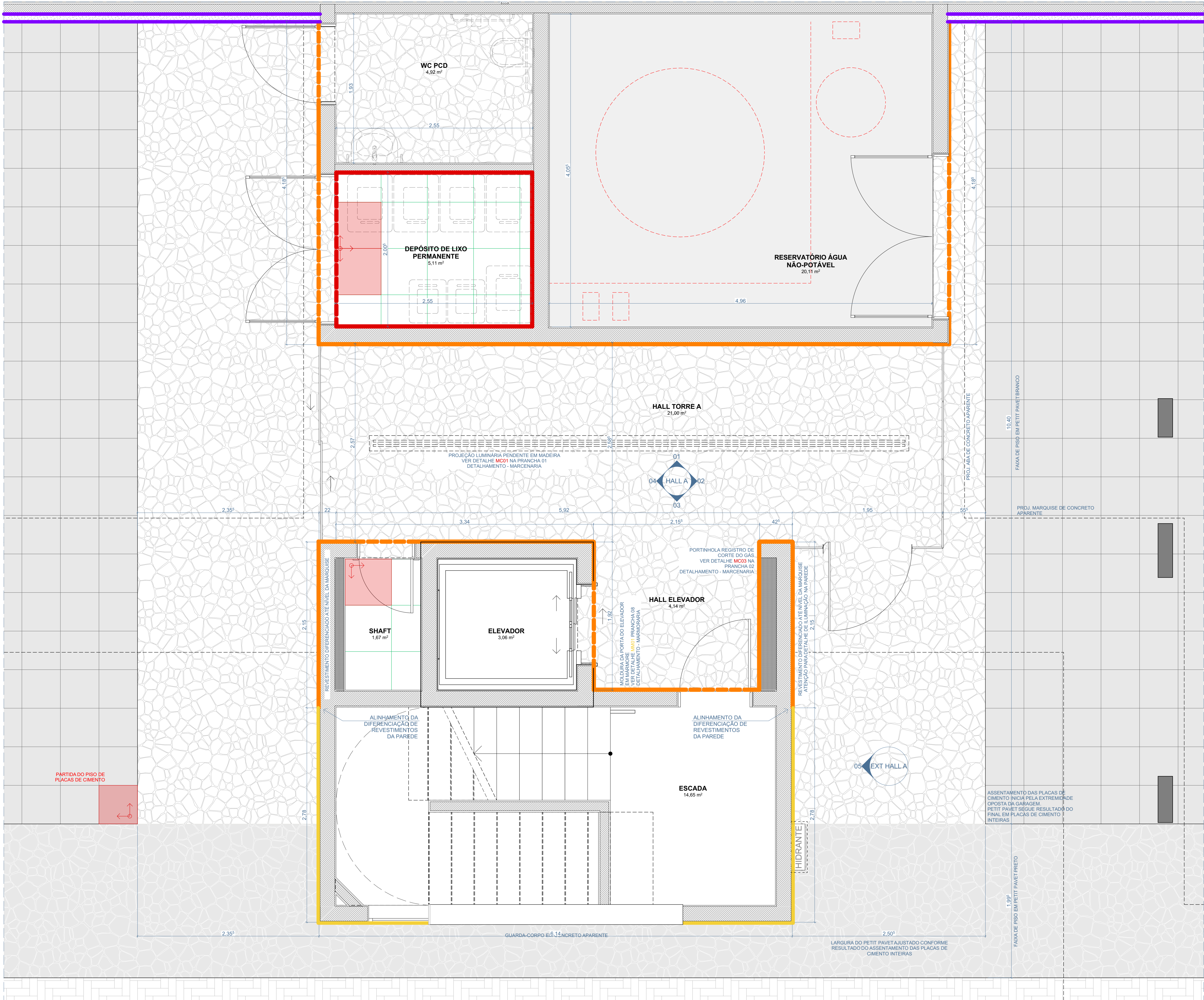
PLANTA BAIXA - HALL A ESCALA 1:25
