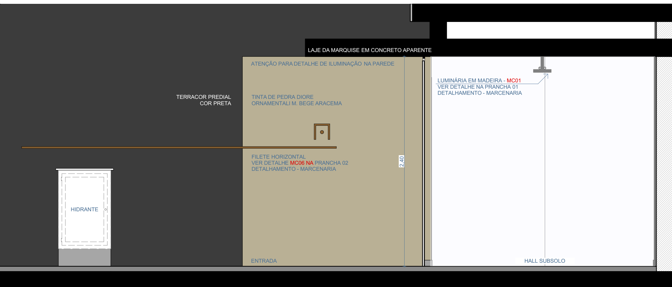
05 - VISTA EXTERNA DO HALL DE ENTRADA ESCALA 1:25
