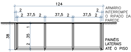
PLANTA BAIXA
