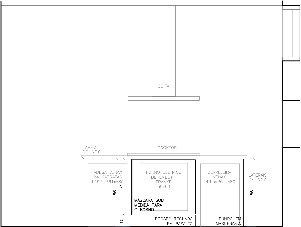
VISTA FRONTAL - ILHA
