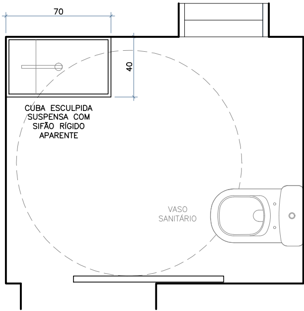
PLANTA BAIXA
