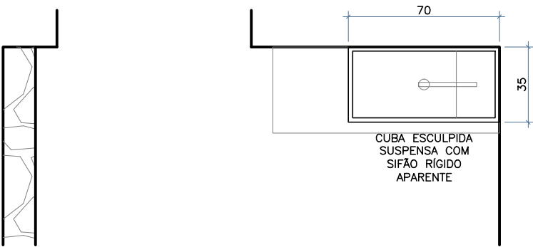
PLANTA BAIXA
