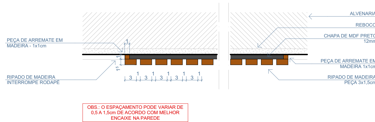
PLANTA BAIXA
