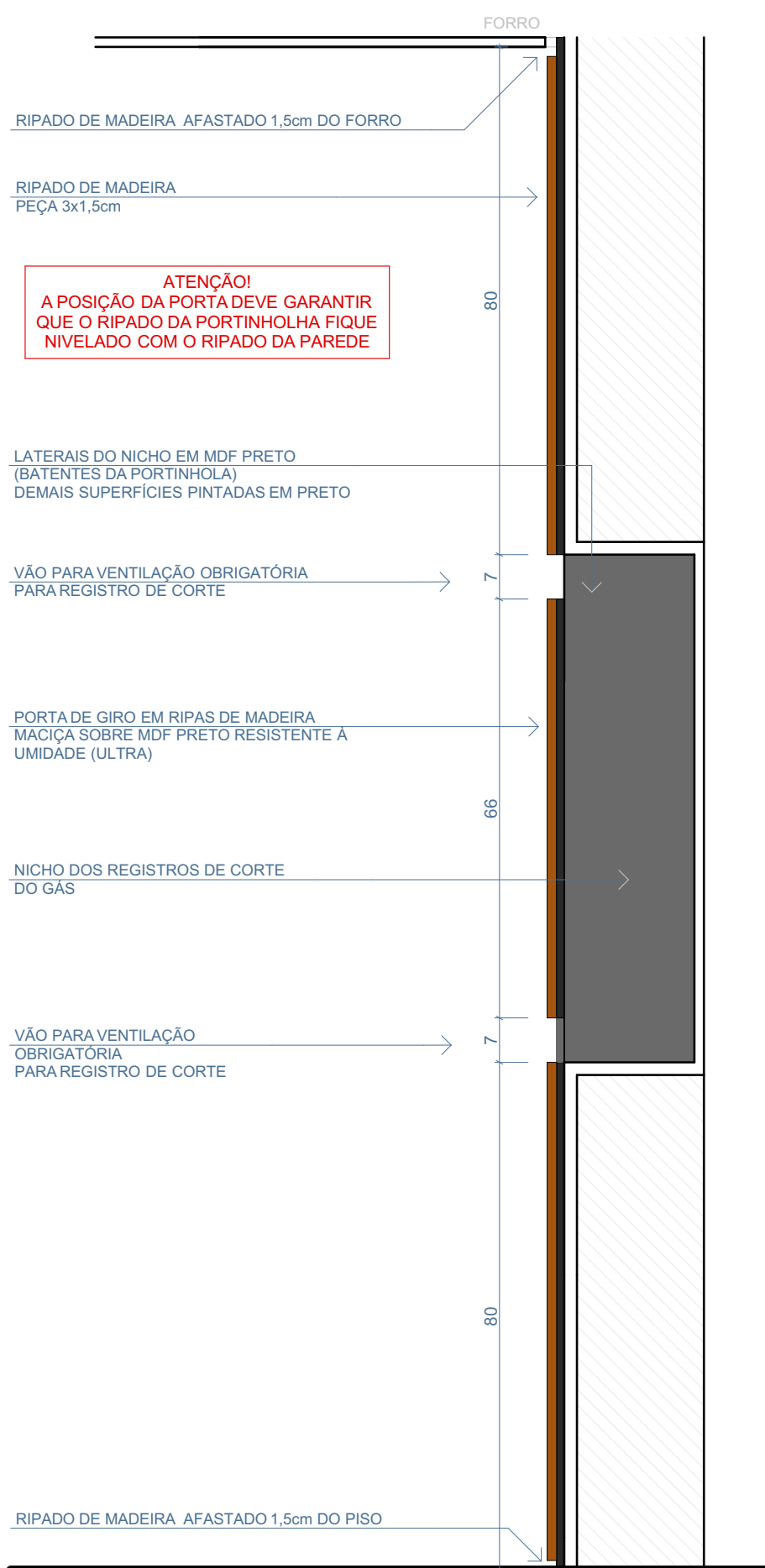
CORTE
