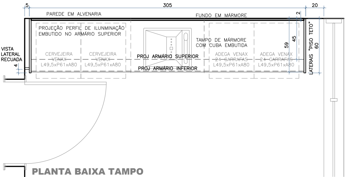
PLANTA BAIXA TAMPO
