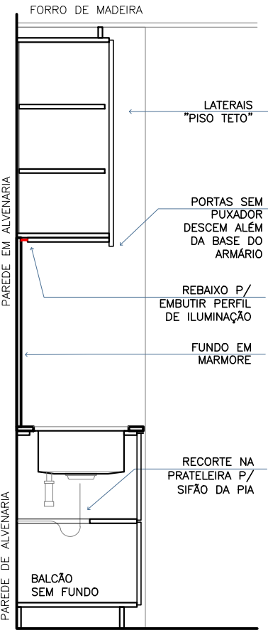
CORTE CUBA
