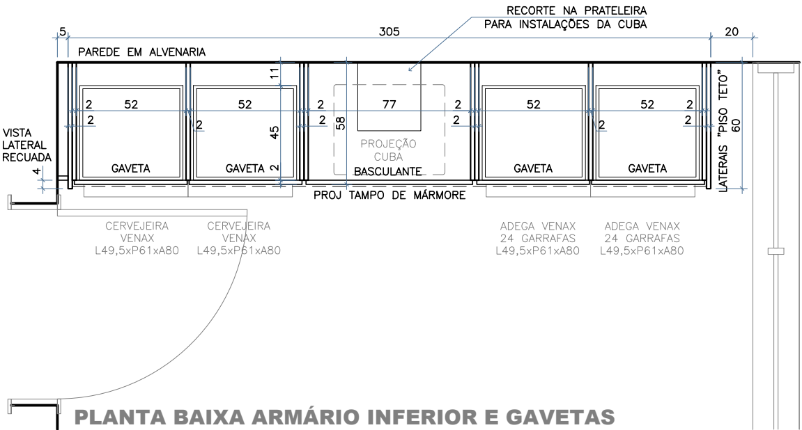
PLANTA BAIXA ARMÁRIO INFERIOR E GAVETAS
