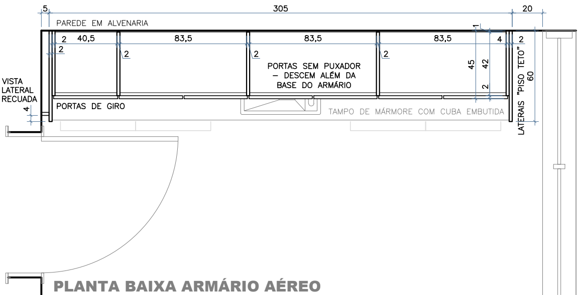
PLANTA BAIXA ARMÁRIO AÉREO
