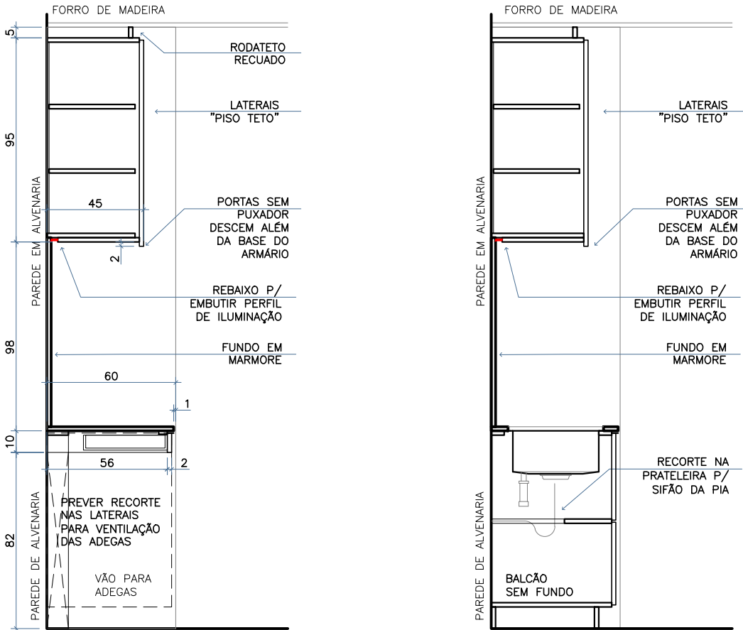
CORTE ESPAÇO CERVEJEIRA
