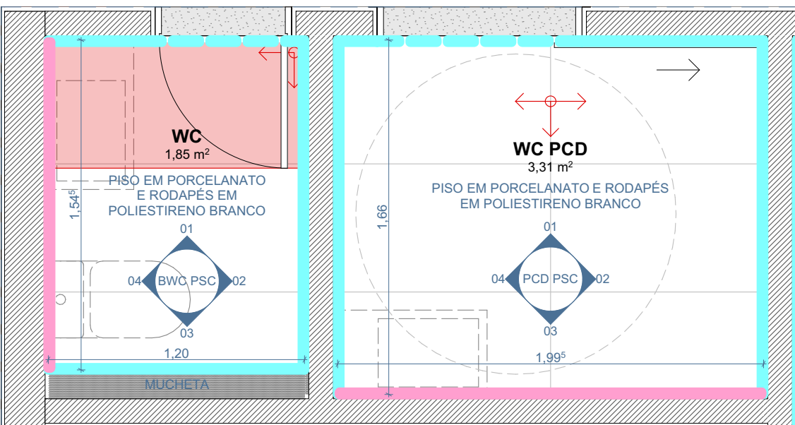
PLANTA BAIXA ESCALA 1:25
