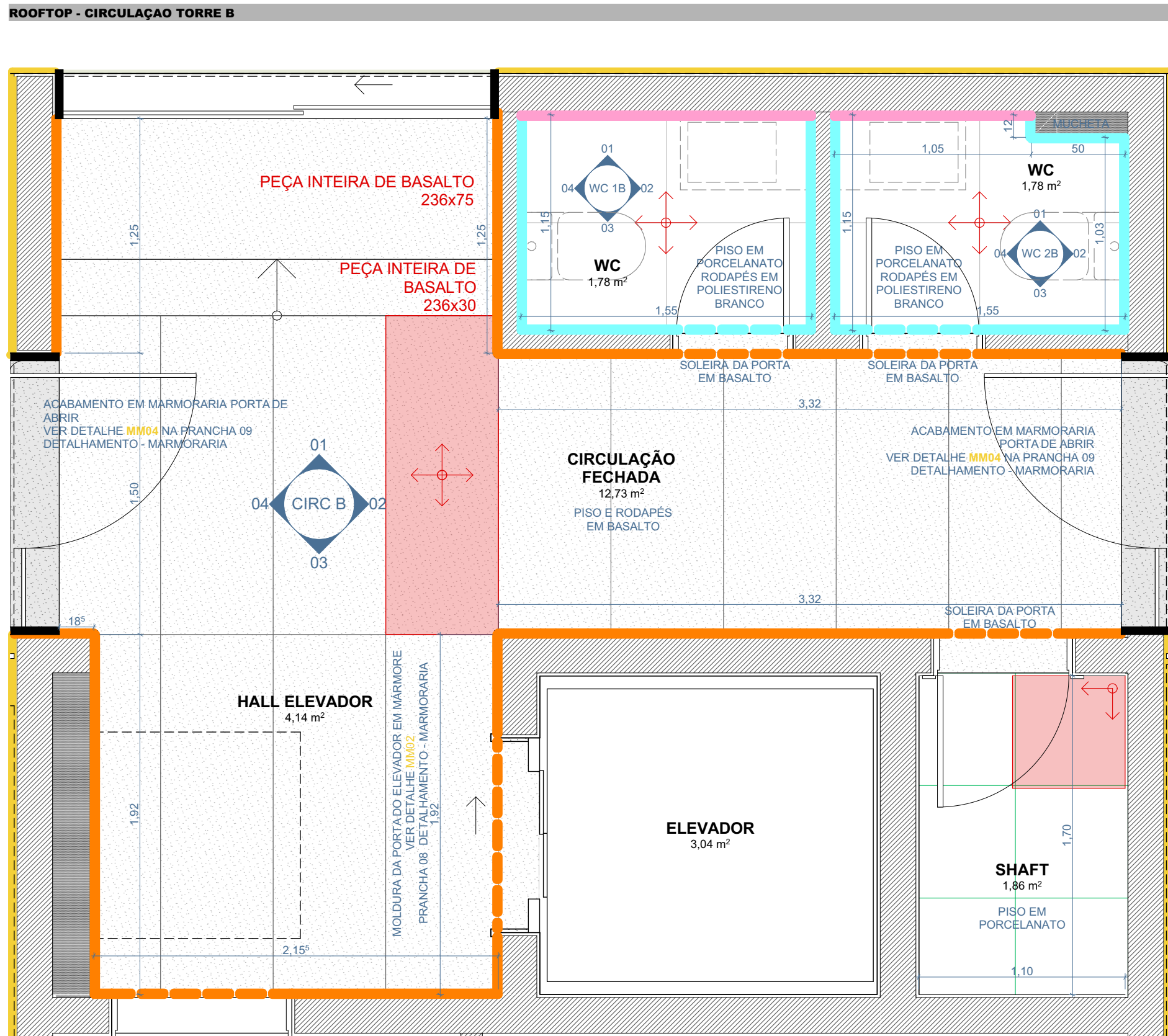
PLANTA BAIXA ESCALA 1:25
