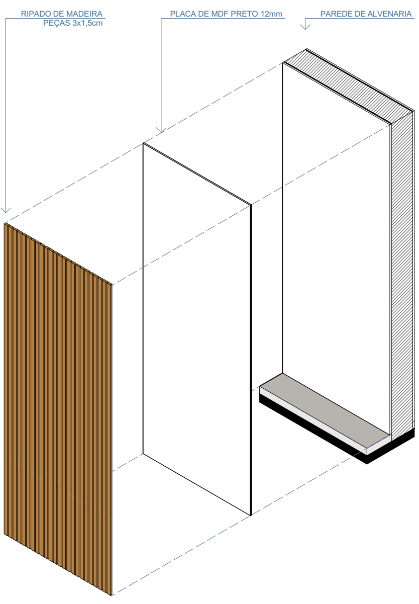
ISOMÉTRICA - RIPADO
