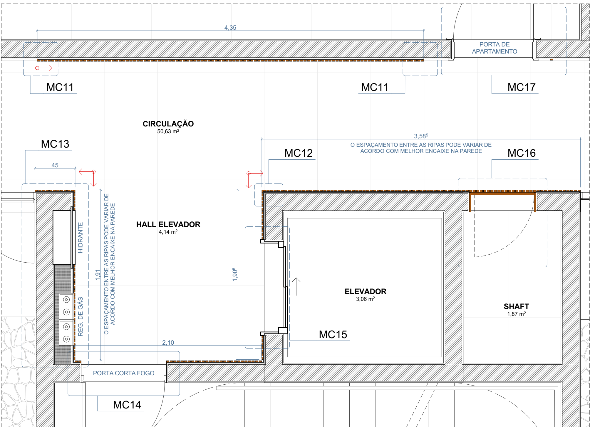
P.BAIXA HALL DOS ELEVADORES - PAGINAÇÃO E INDICAÇÃO DE DETALHES ESCALA 1:25
