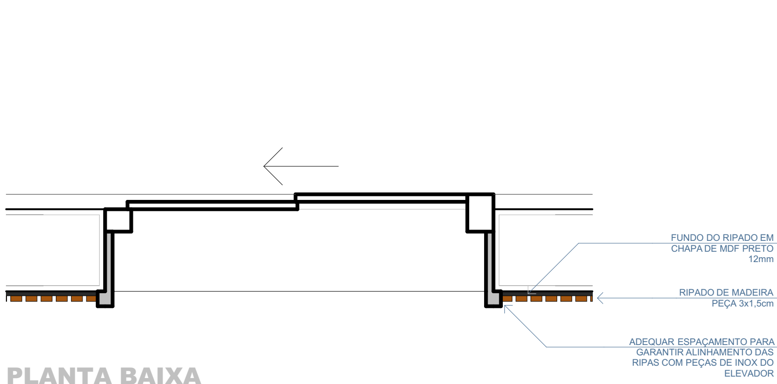
PLANTA BAIXA
