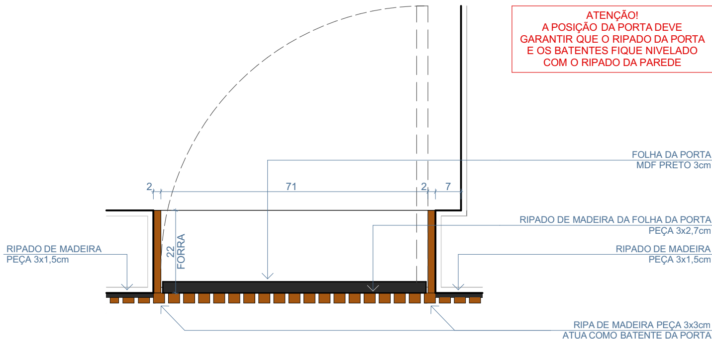
PLANTA BAIXA
