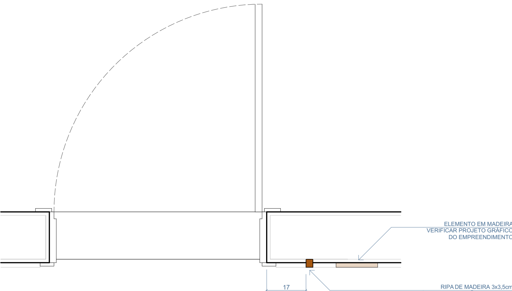
PLANTA BAIXA
