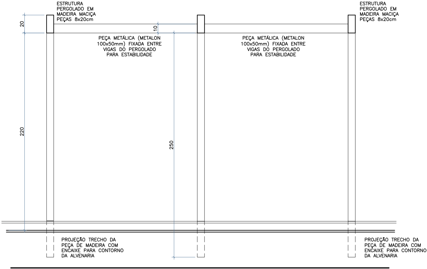
CORTE
