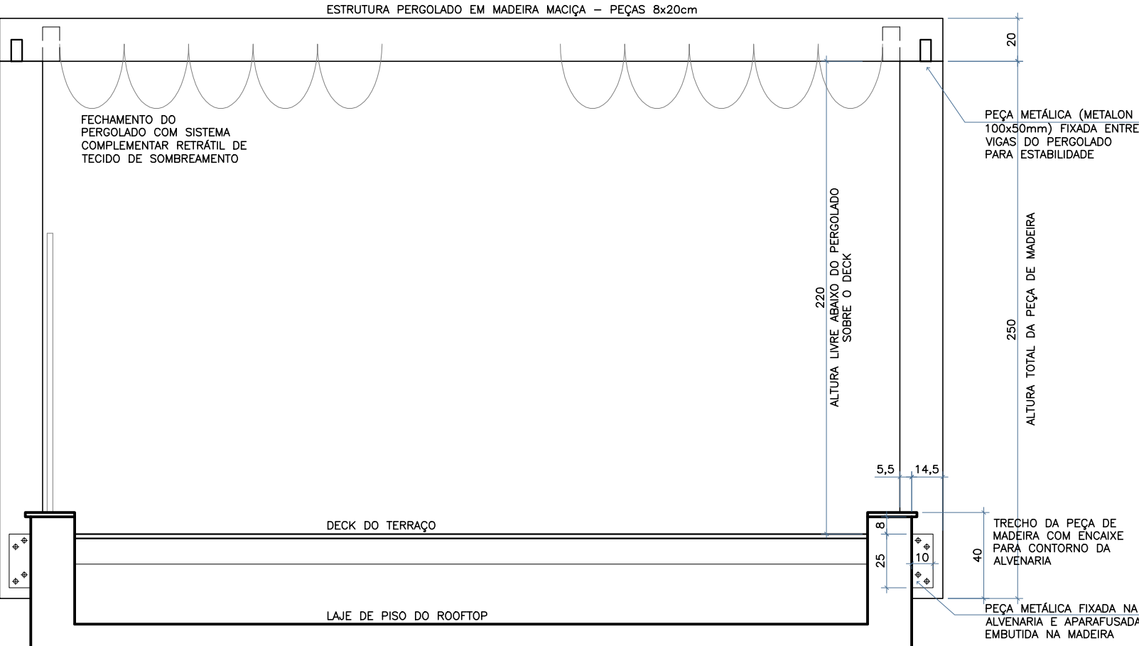
VISTA LATERAL
