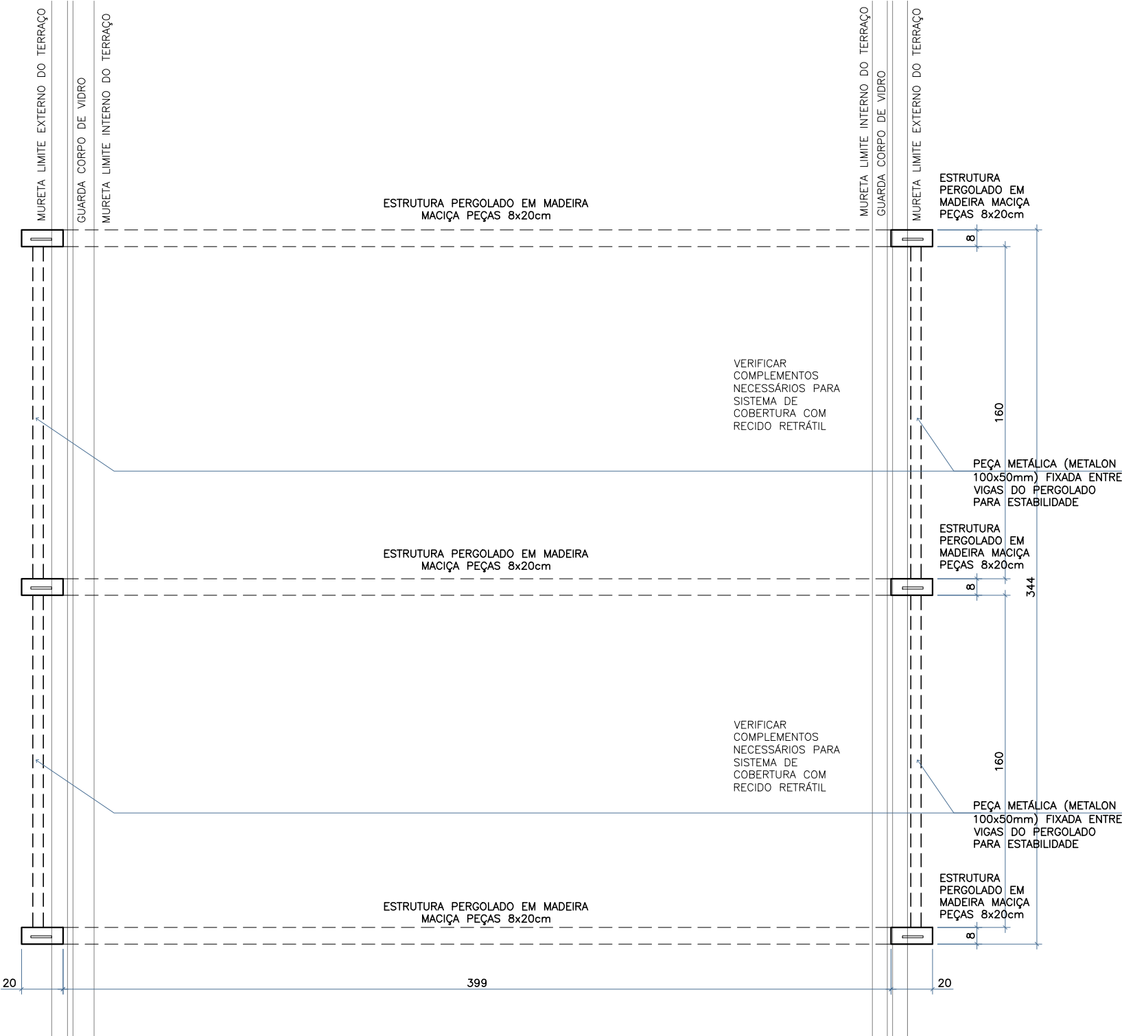
PLANTA BAIXA
