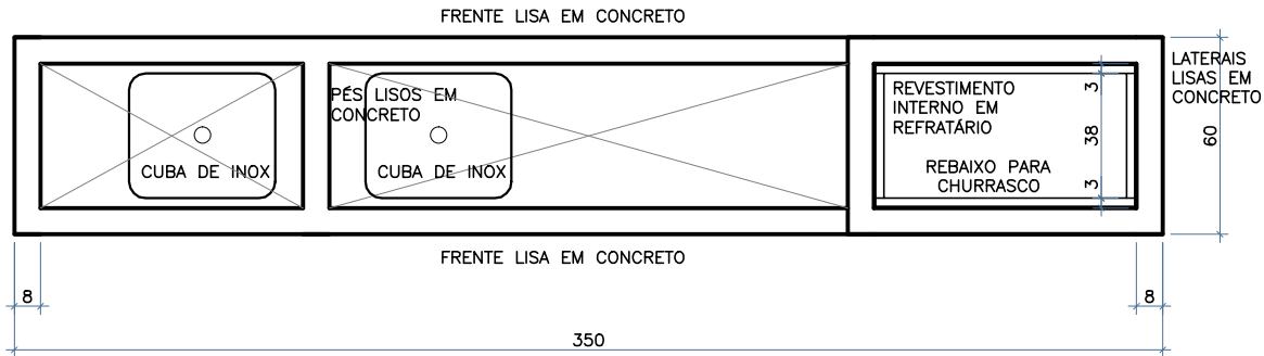
PLANTA BAIXA NÍVEL DECK (PISO ACABADO)
