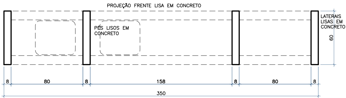
PLANTA BAIXA NÍVEL LAJE (OSSO)
