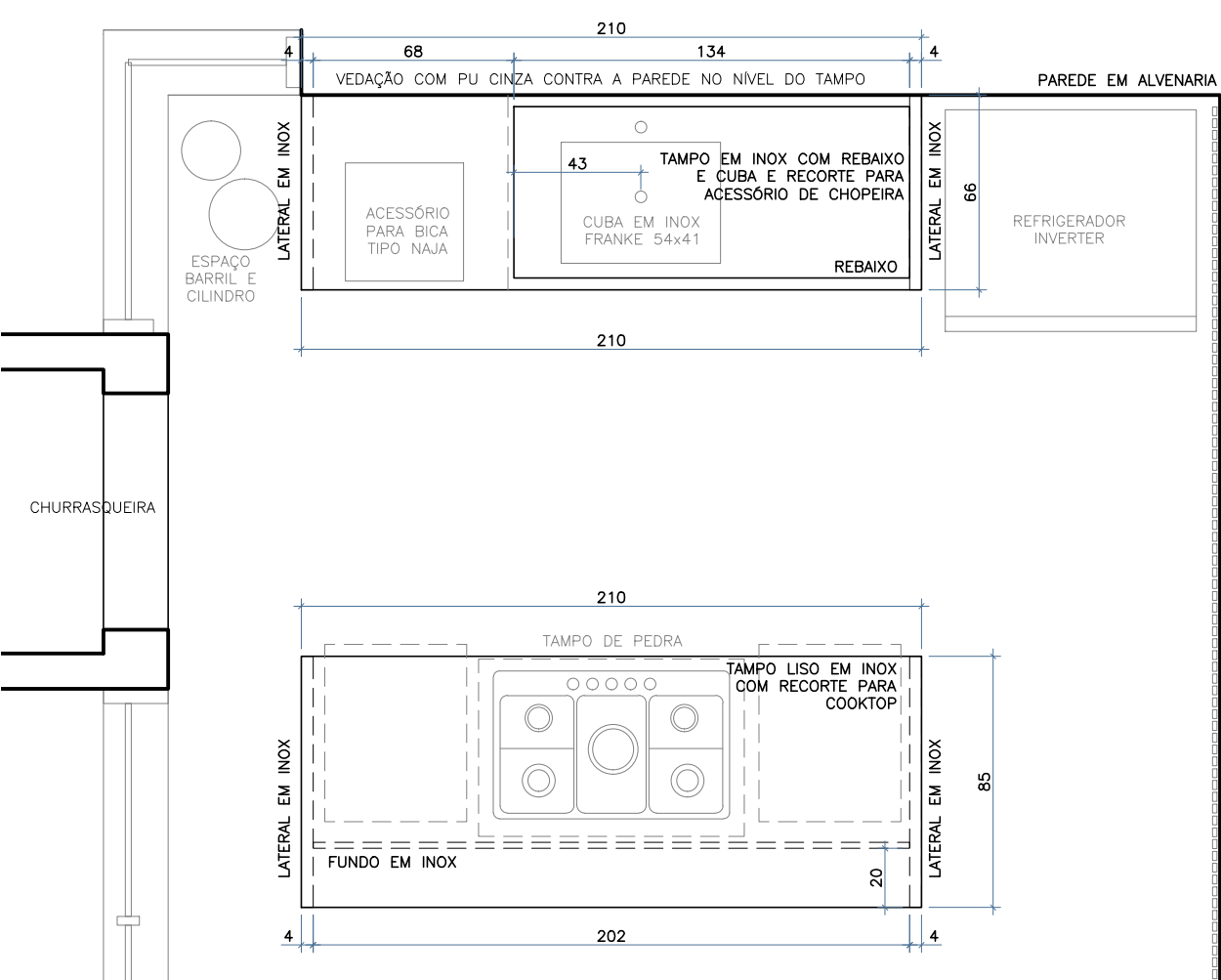
VISTA SUPERIOR
