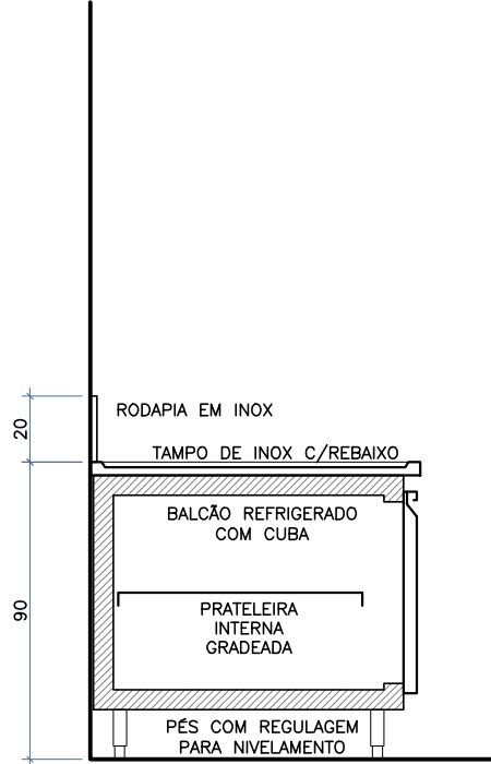
CORTE 01
