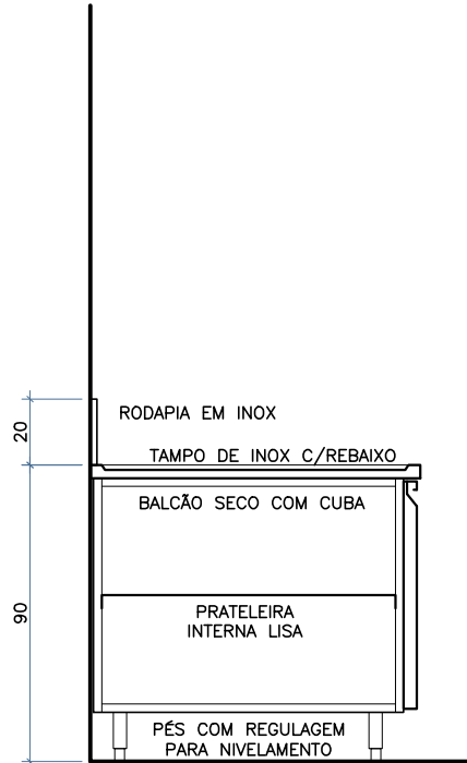
CORTE 01
