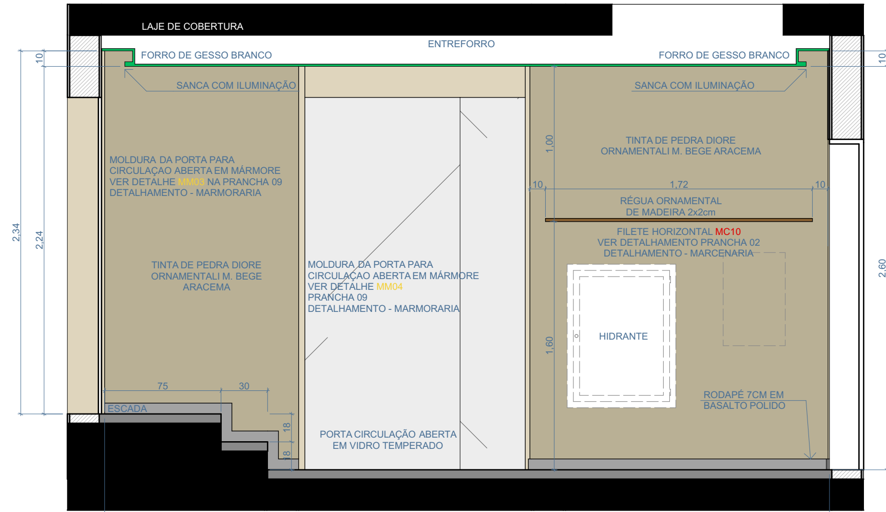
02 ESCALA 1:25
