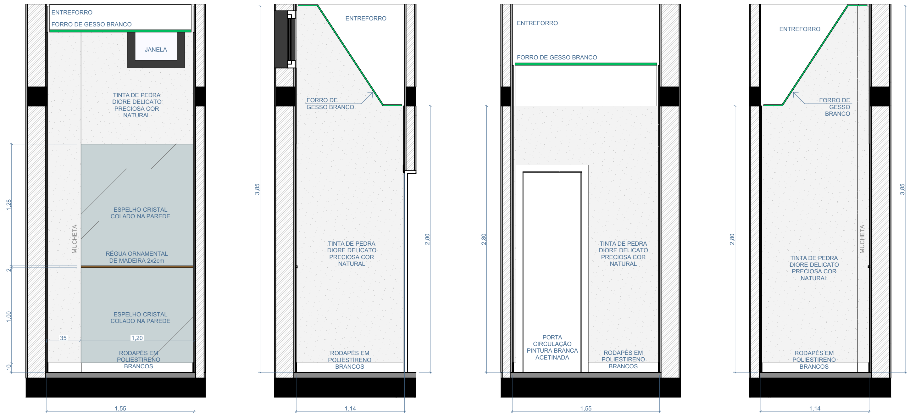
01 ESCALA 1:25
