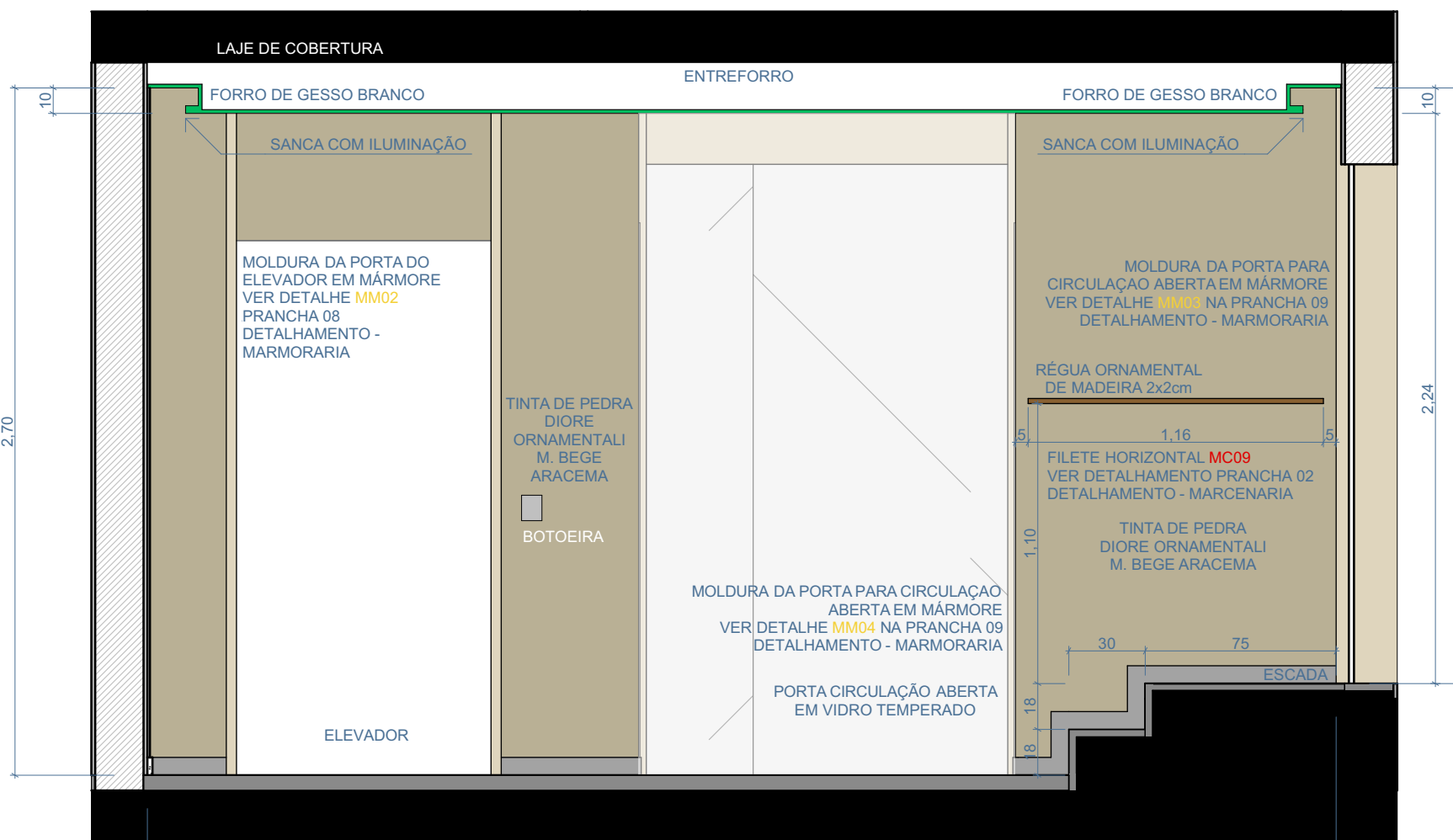
04 ESCALA 1:25
