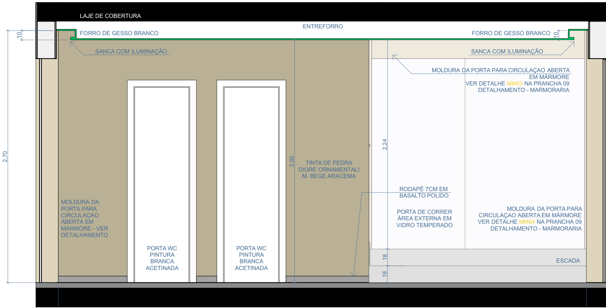
01 ESCALA 1:25
