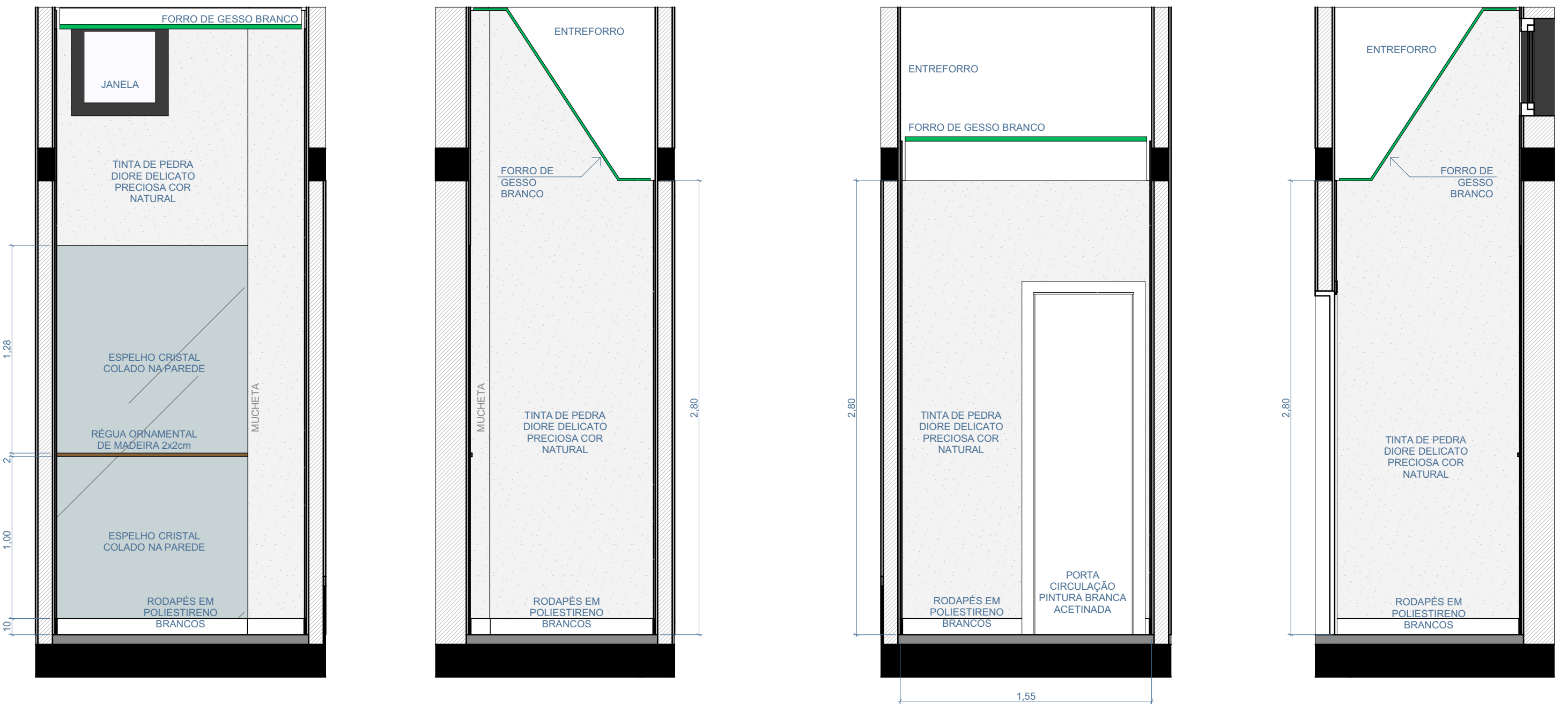
01 ESCALA 1:25
