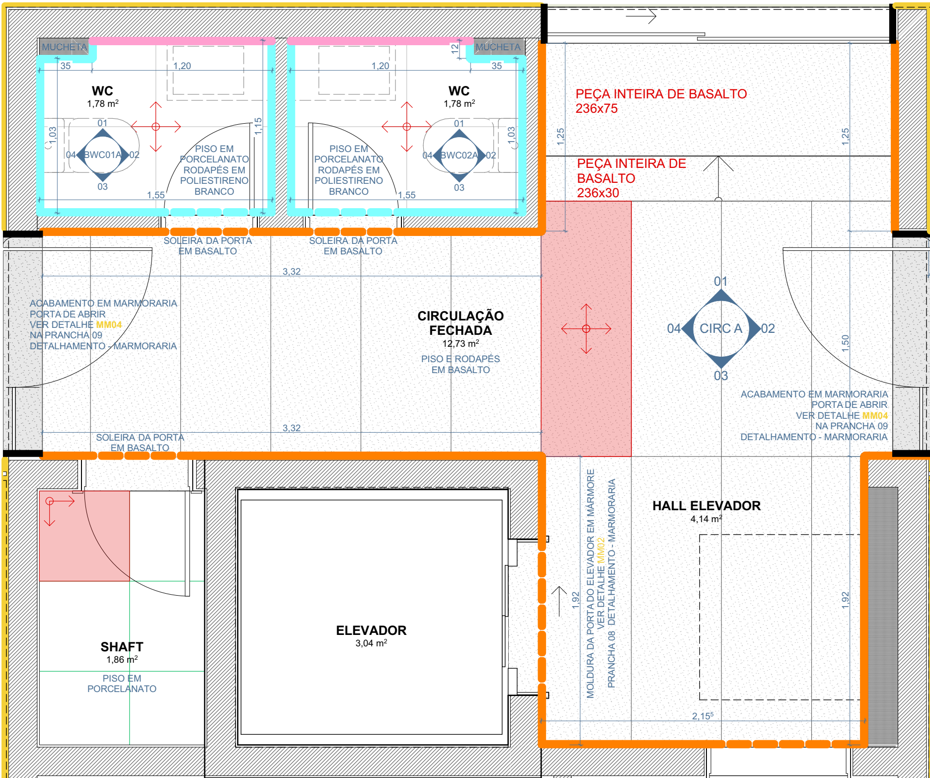
PLANTA BAIXA ESCALA 1:25
