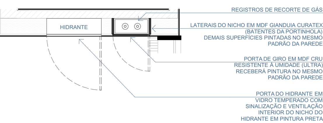
PLANTA BAIXA
