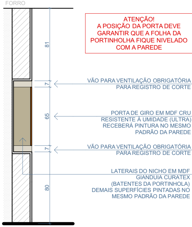
CORTE
