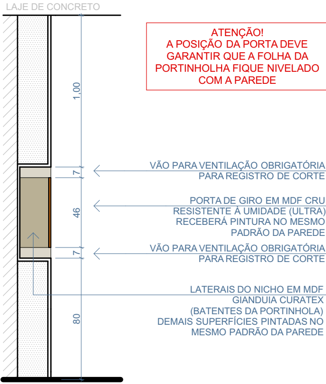
CORTE
