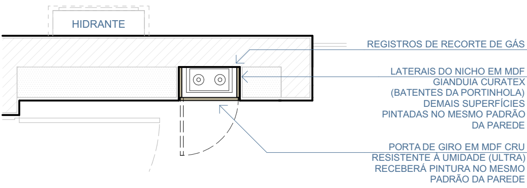
PLANTA BAIXA
