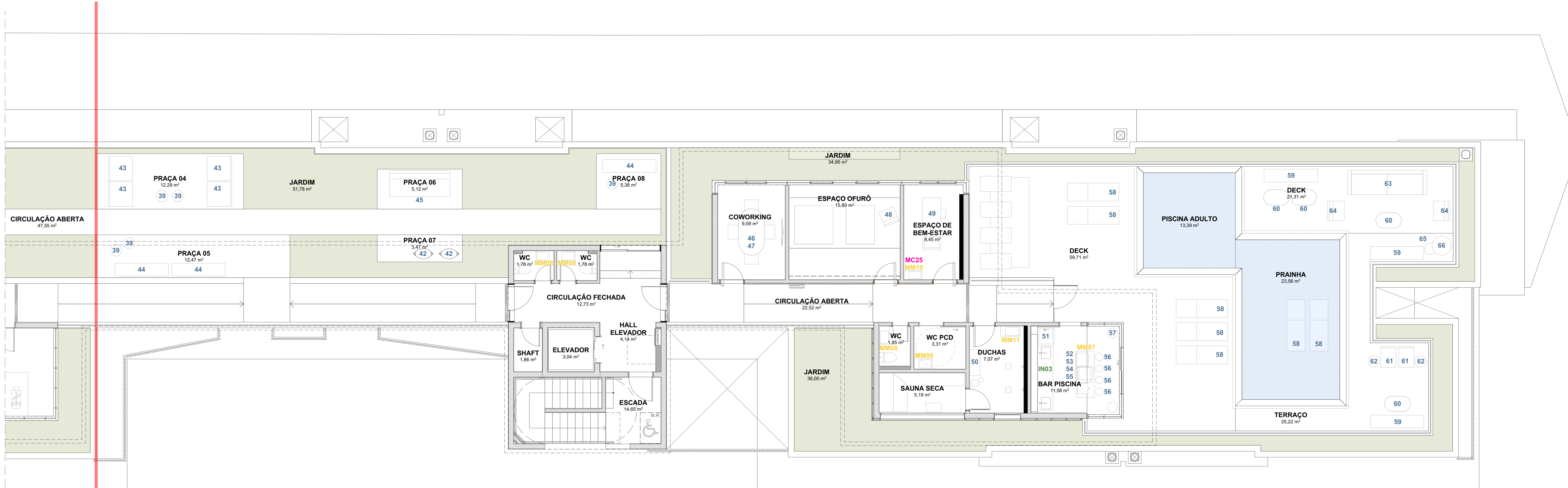
PLANTA BAIXA ESCALA 1:75 TRECHO 1
