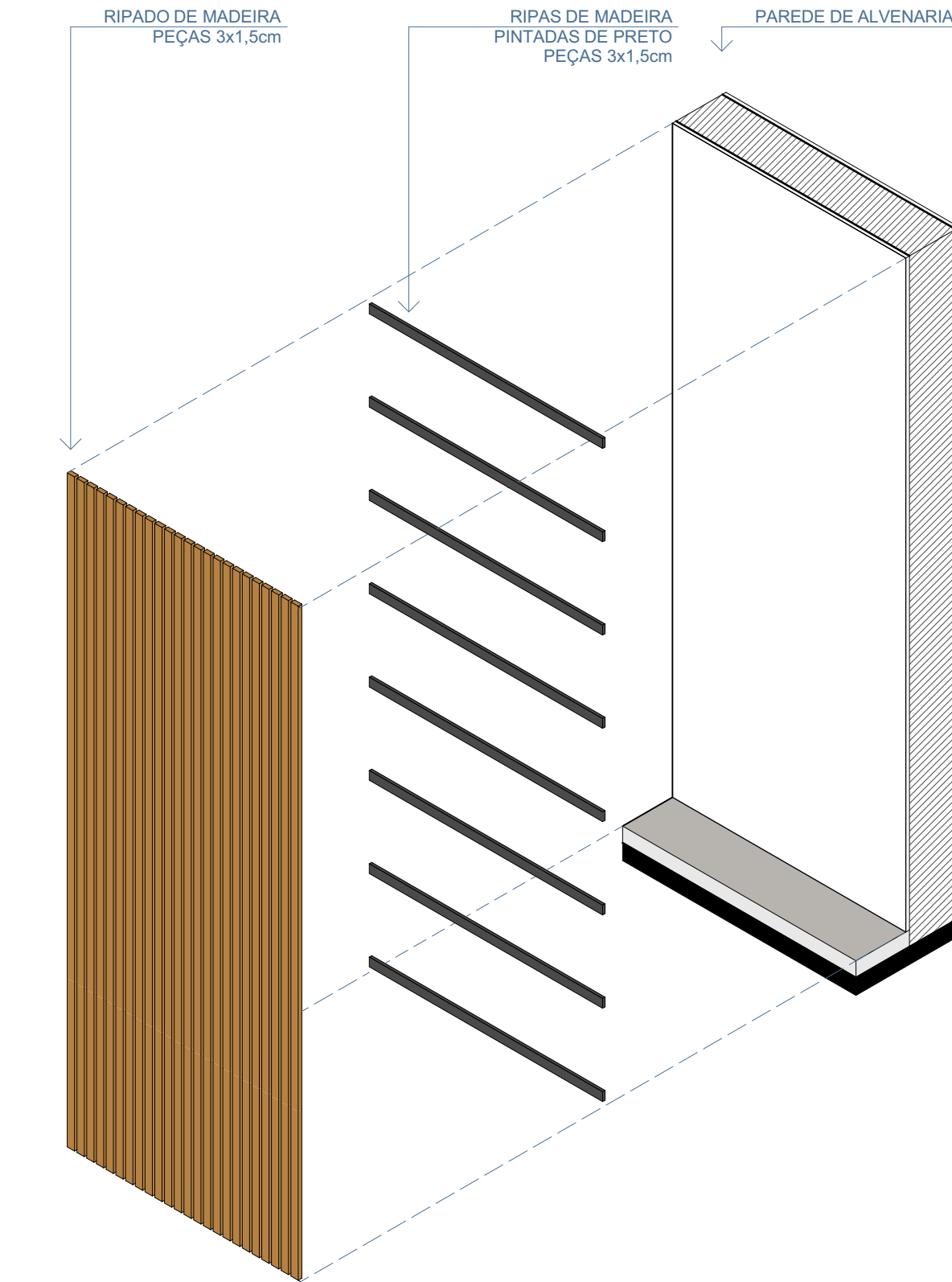
ISOMÉTRICA - RIPADO
