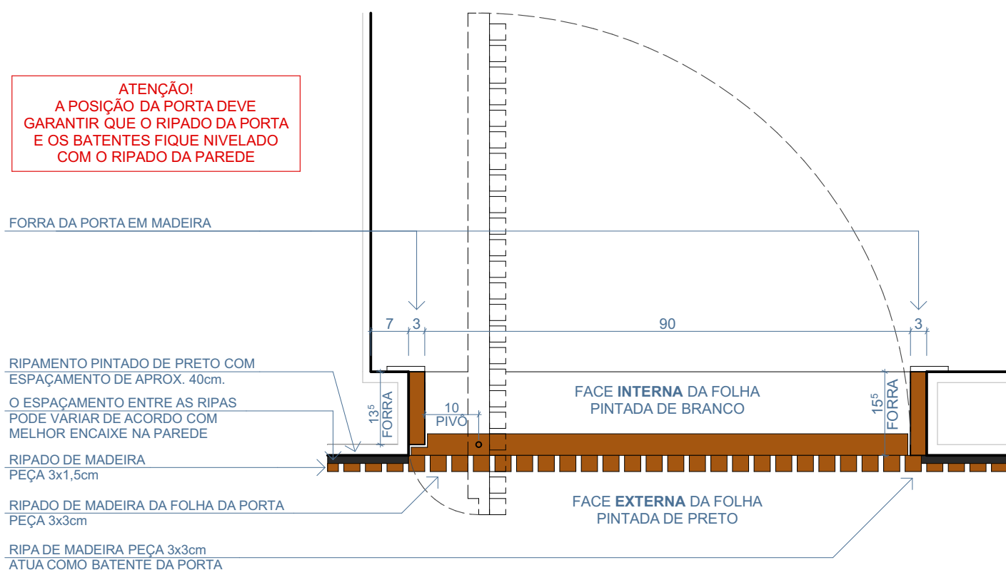
PLANTA BAIXA
