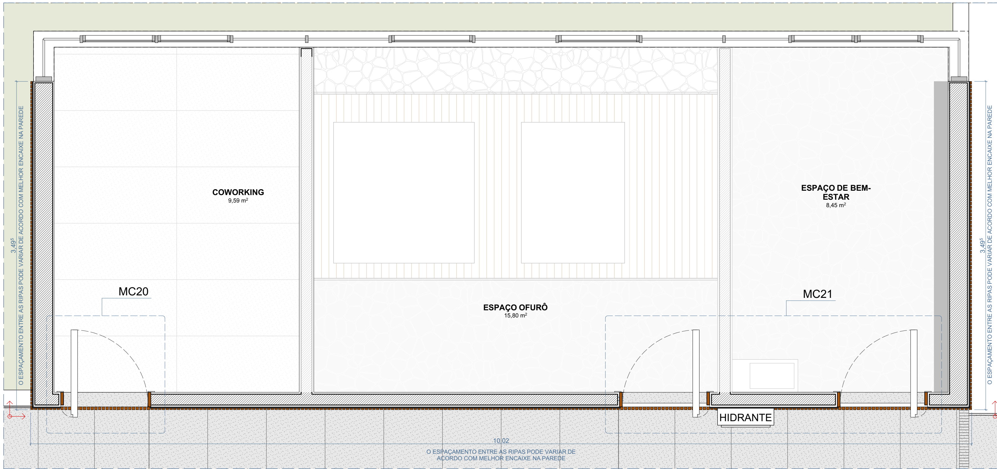
PLANTA BAIXA CIRCULAÇÃO ROOFTOP - PAGINAÇÃO DO RIPADO E INDICAÇÃO DE DETALHES ESCALA 1:25
