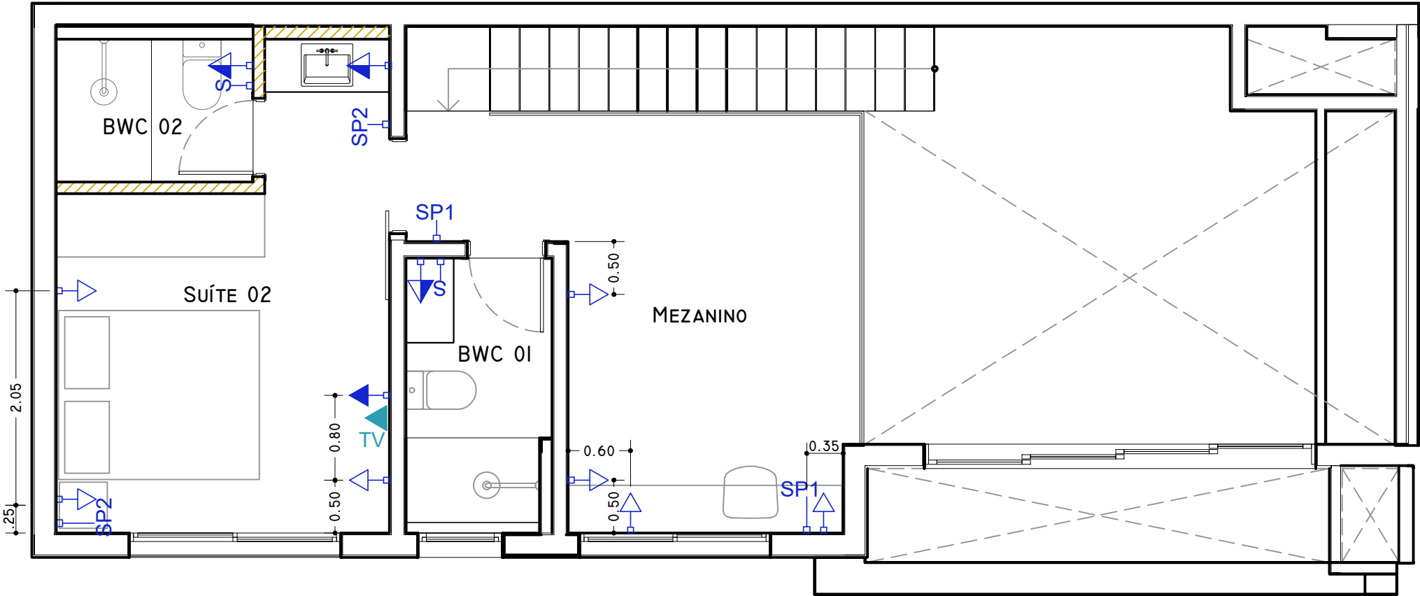
PLANTA BAIXA - PONTOS ELÉTRICA UNIDADE 204 AP 1 prop. LUIS FERNANDO M. MAX
