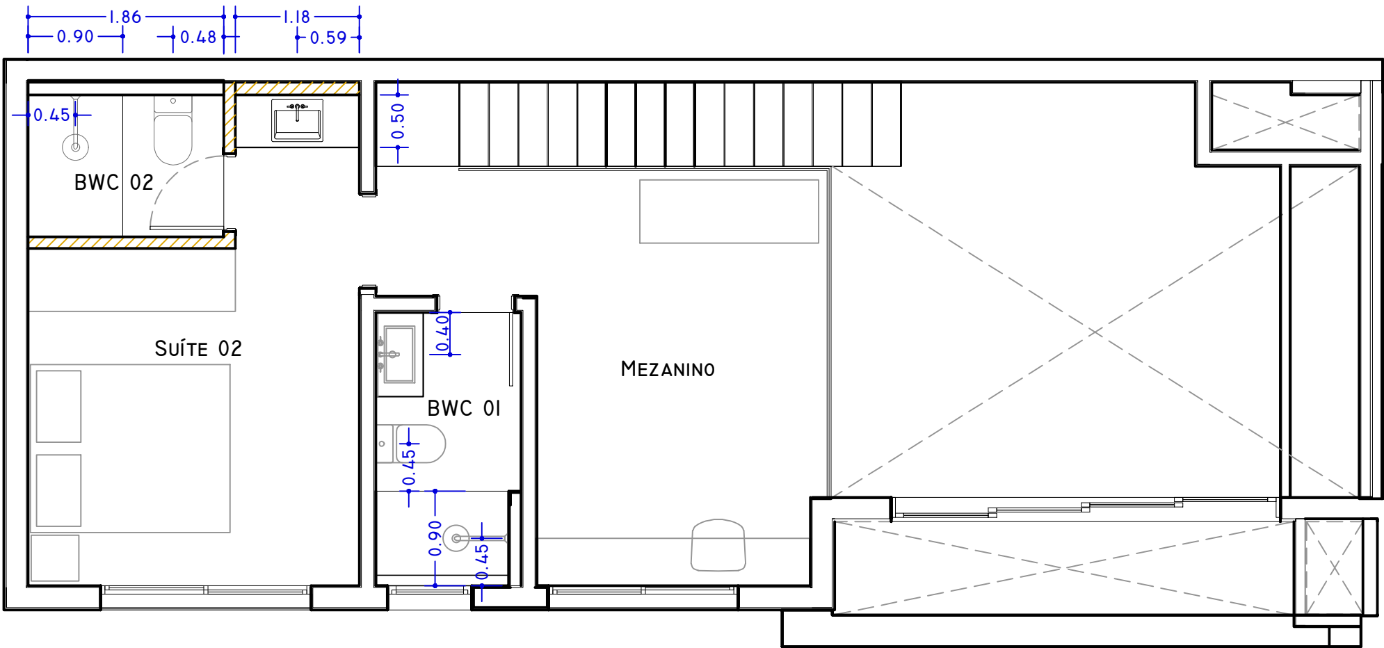
PLANTA BAIXA - PONTOS HIDRÁULICA UNIDADE 204 AP 1 prop. LUIS FERNANDO M. MAX
