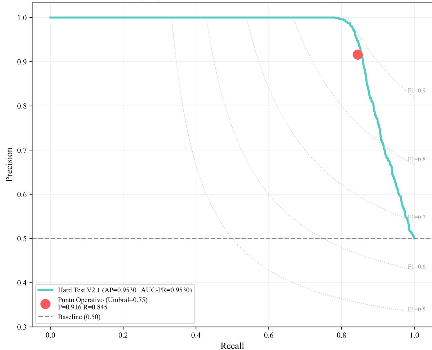
Hard Test V2.1 - Curva de Precision-Recall (Target=5 Taranis excluido del entrenamiento)
