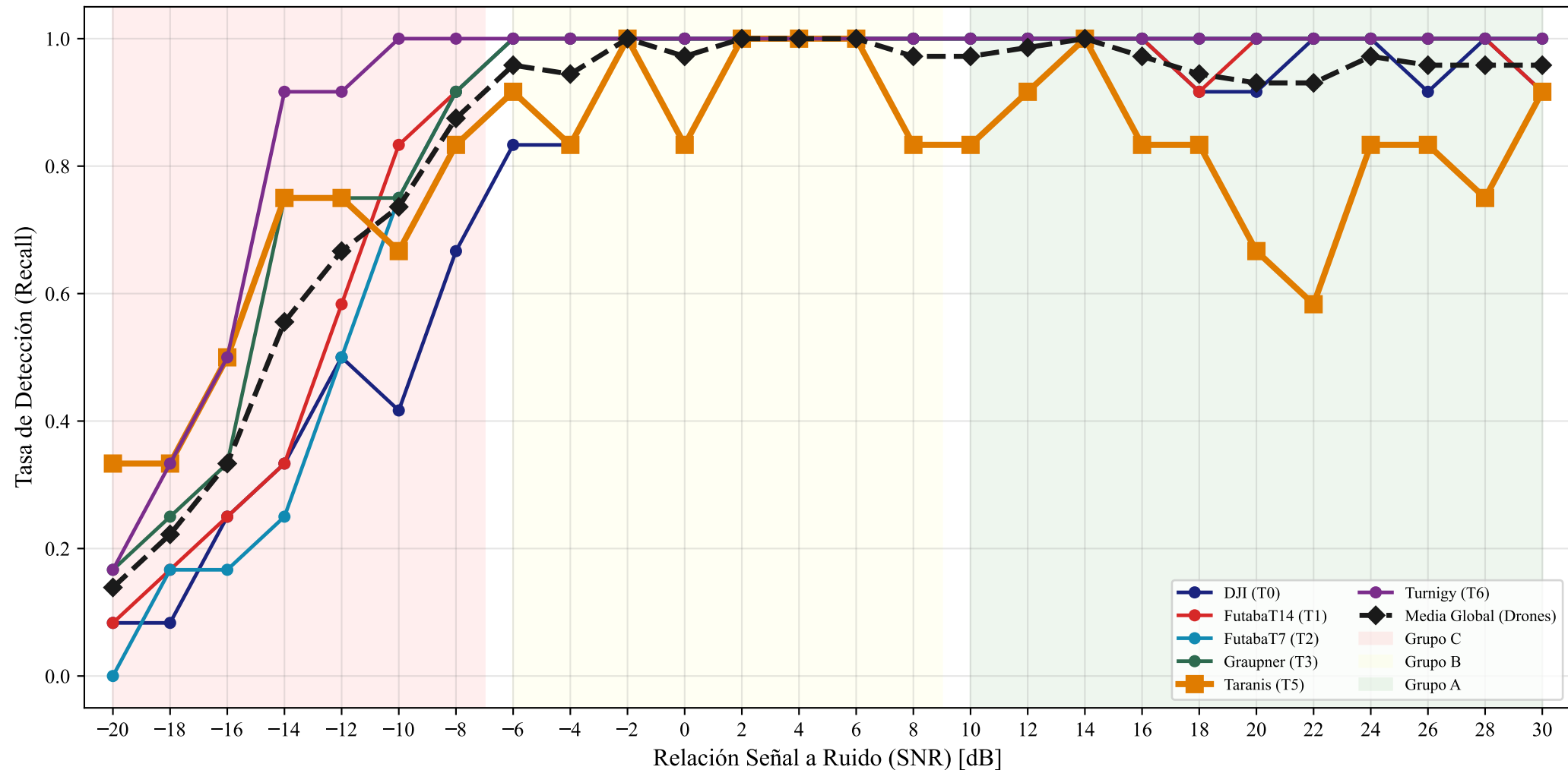
Tasa de Detección por Emisor RF en función de la SNR Taranis T5 = HELD-OUT, nunca visto durante el entrenamiento
