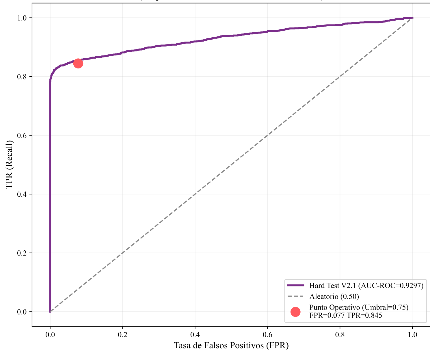
Hard Test V2.1 - Curva ROC (Target=5 Taranis excluido del entrenamiento)
