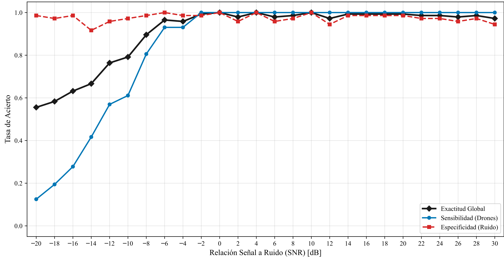
Exactitud del Clasificador por Nivel de SNR (Umbral=0.91)
