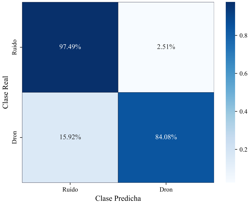
Matriz de Confusión sobre Test Ciego (Umbral=0.91)
