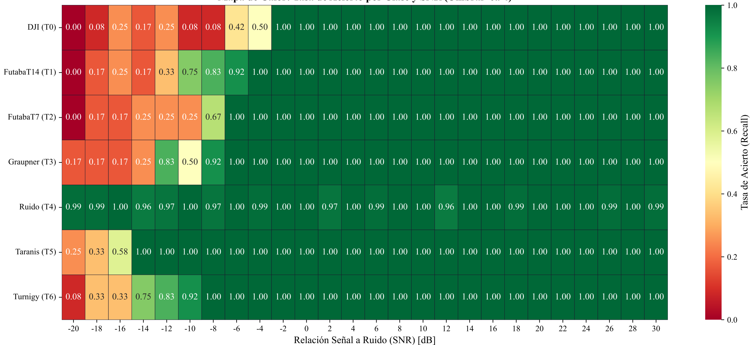
Mapa de Calor: Tasa de Acierto por Clase y SNR (Umbral=0.94)
