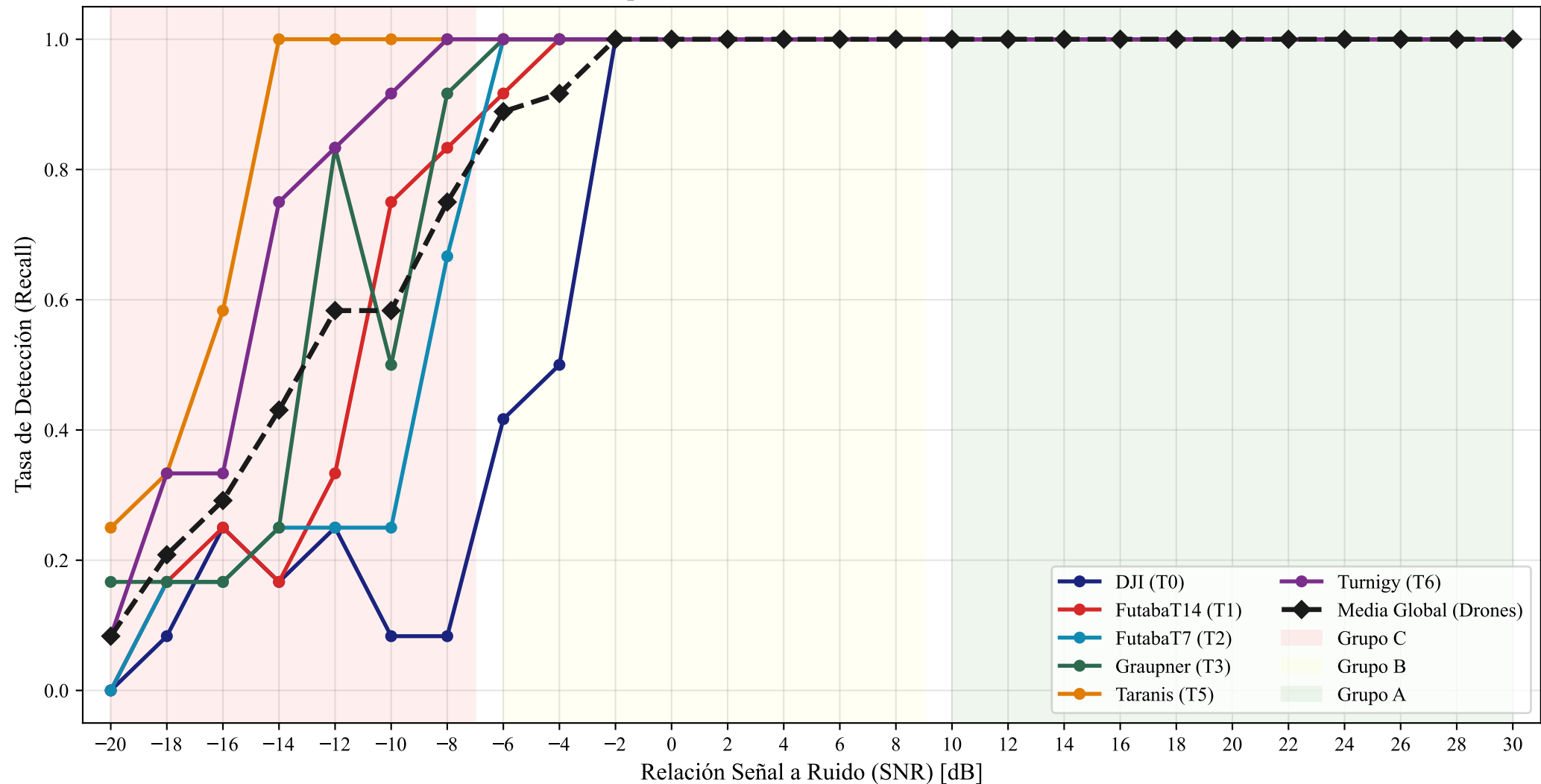
Tasa de Detección por Emisor RF en función de la SNR (Umbral=0.94)
