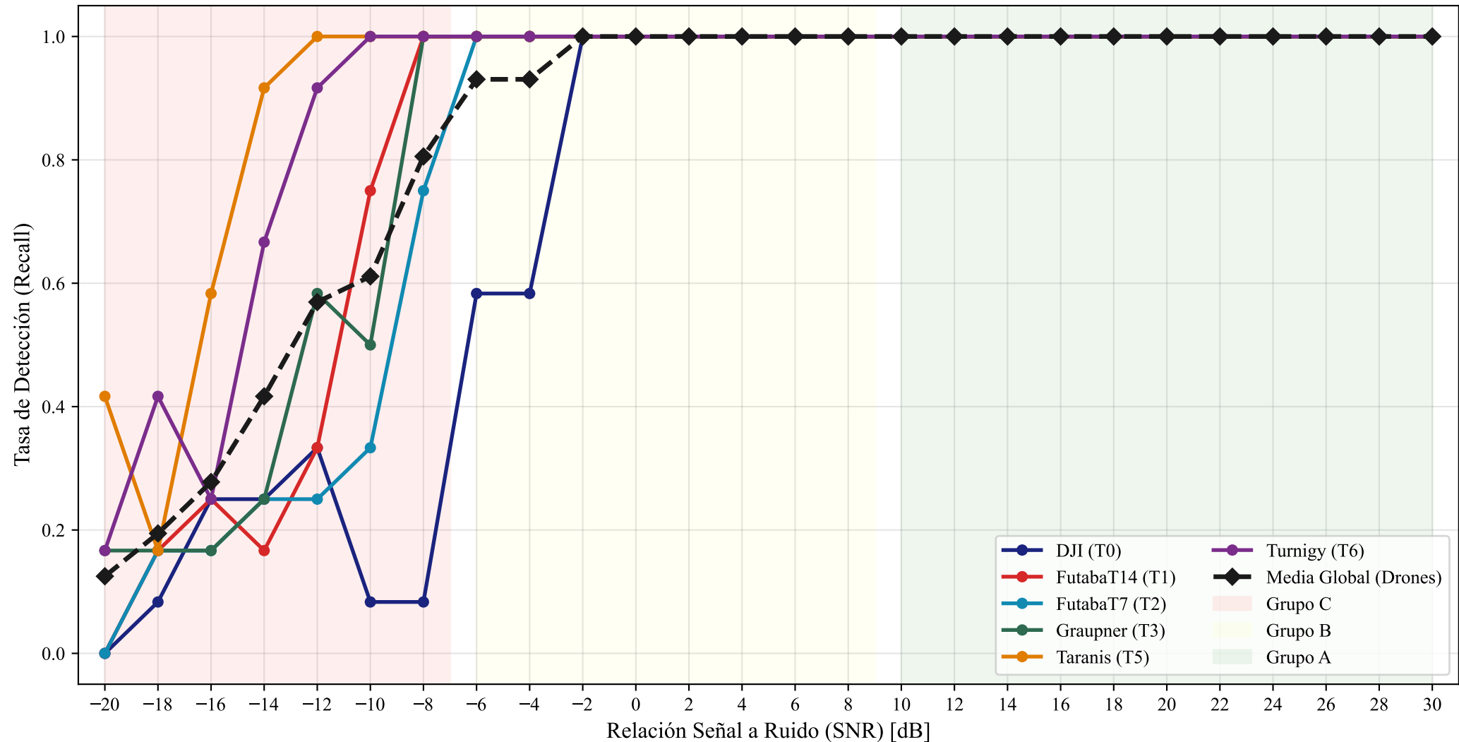
Tasa de Detección por Emisor RF en función de la SNR (Umbral=0.91)
