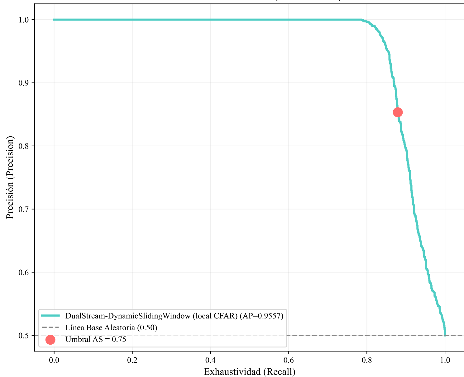
Curva Precision-Recall - Modo Alta Sensibilidad (Umbral=0.75)
