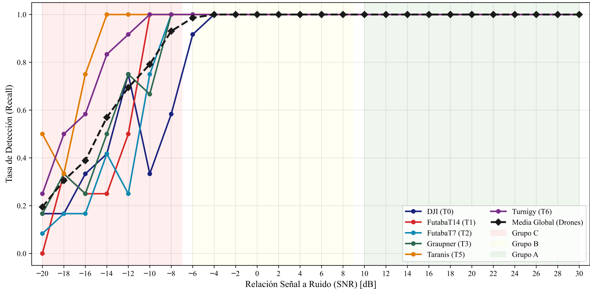
Tasa de Detección por Emisor RF en función de la SNR - Modo Alta Sensibilidad (Umbral=0.75)
