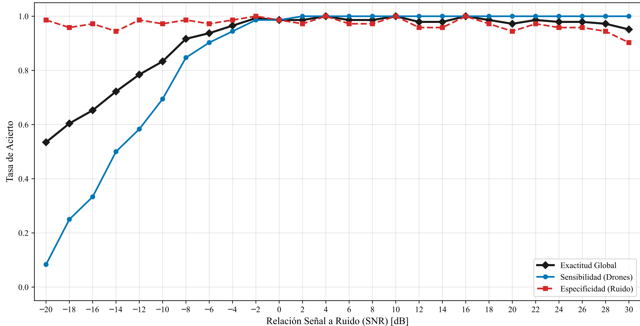
Exactitud del Clasificador por Nivel de SNR (Umbral=0.90)
