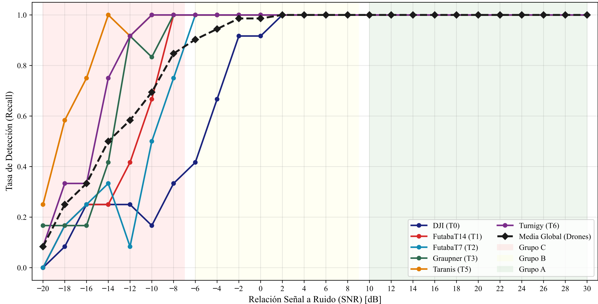
Tasa de Detección por Emisor RF en función de la SNR (Umbral=0.90)
