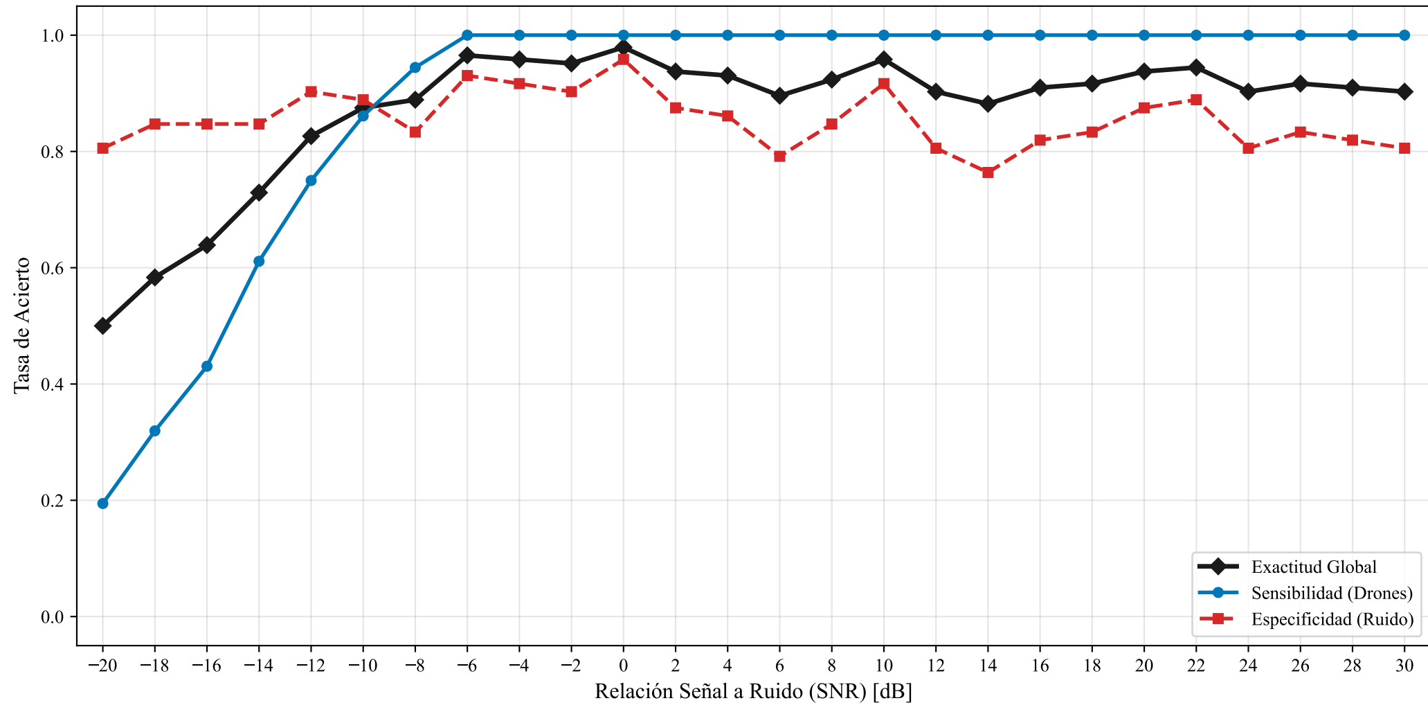
Exactitud del Clasificador por Nivel de SNR - Modo Alta Sensibilidad (Umbral=0.75)
