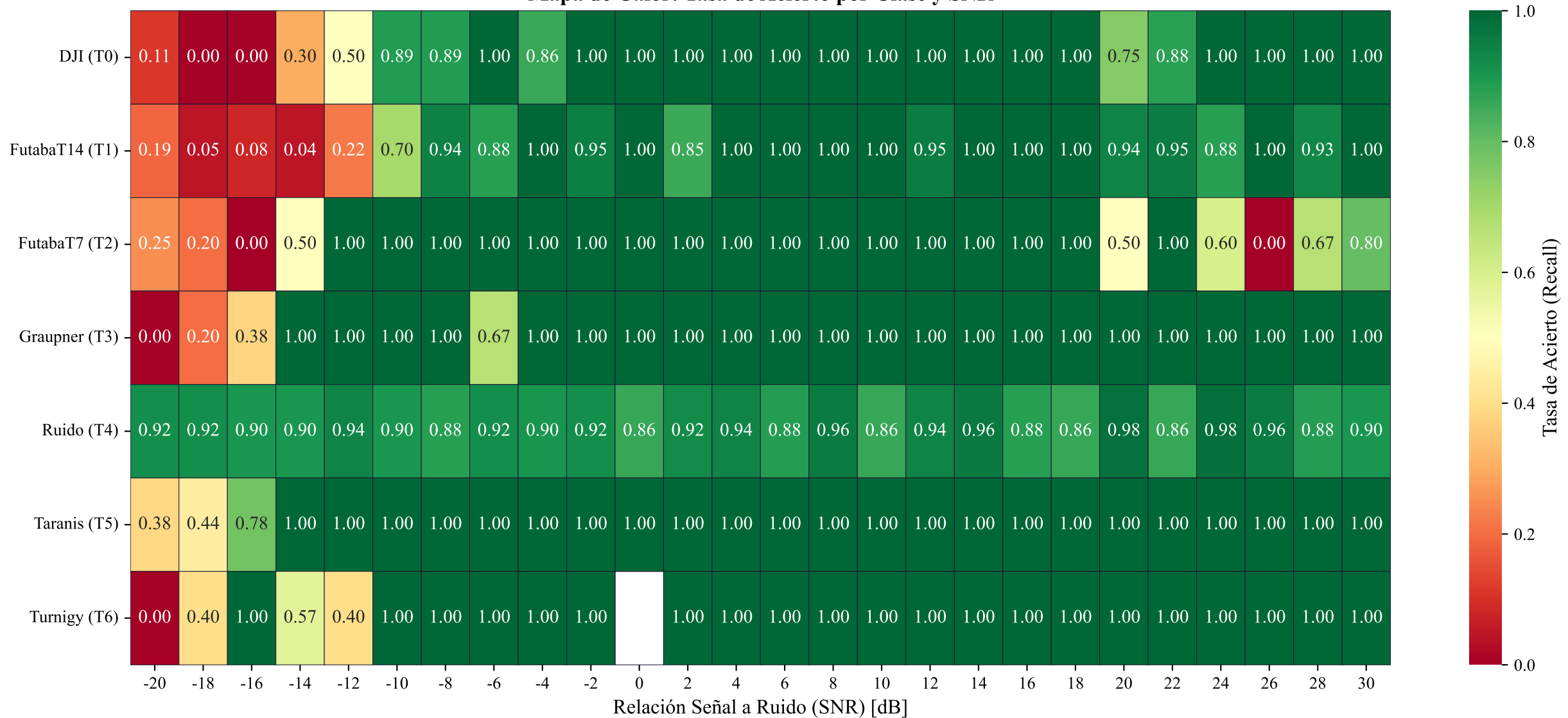
Mapa de Calor: Tasa de Acierto por Clase y SNR
