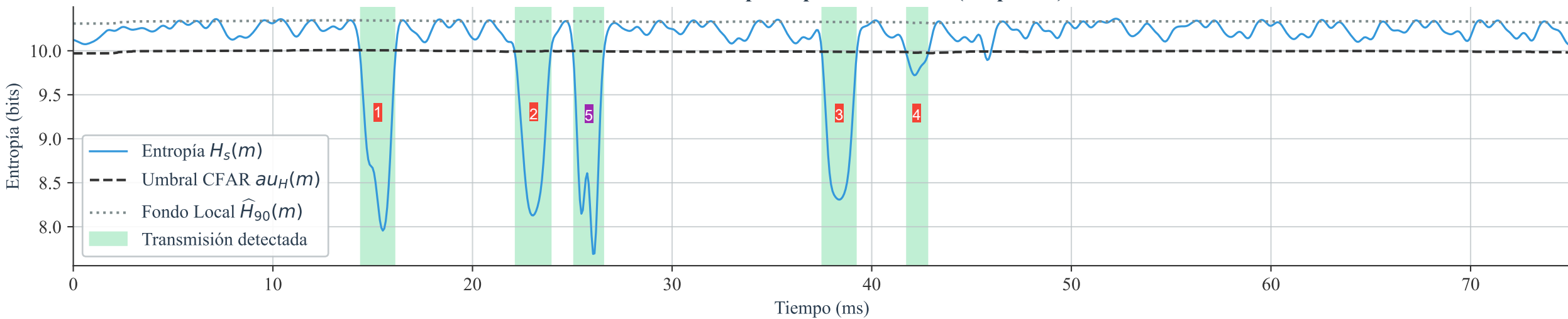
Detector de Entropía Espectral + CFAR (Propuesto)
