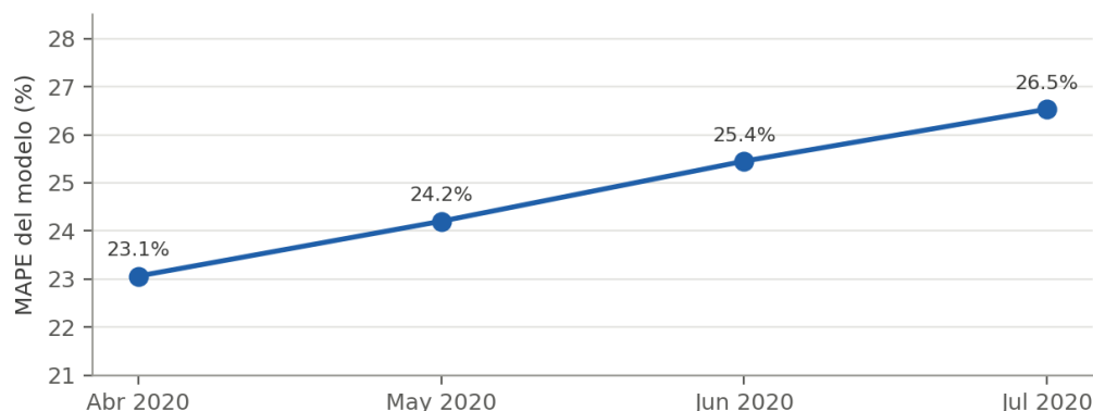
Figura 5. Error relativo del modelo por mes de publicación, sobre el conjunto de evaluación (abril a julio de 2020).
