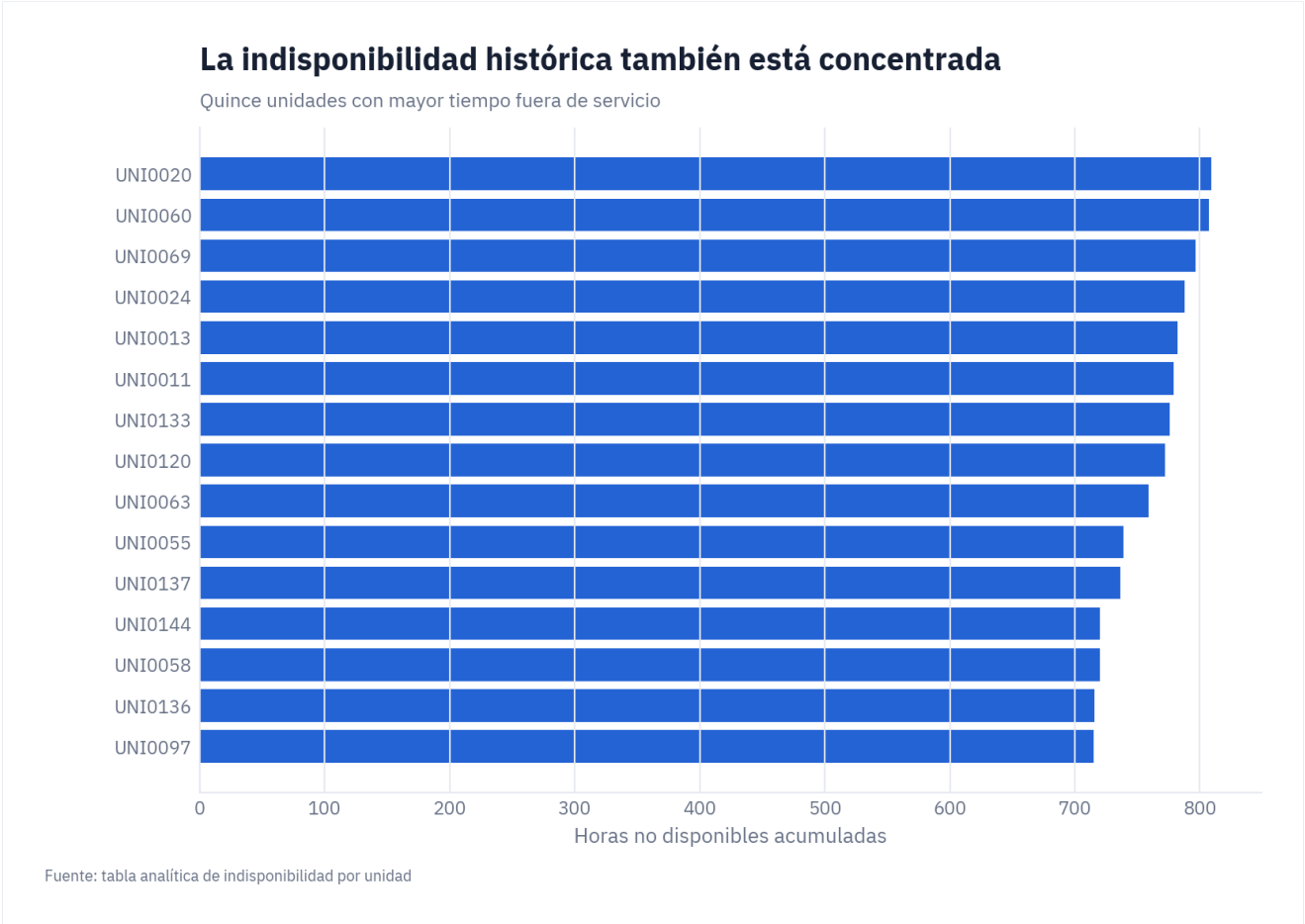
Figura. Un conjunto reducido de unidades concentra una proporción desproporcionada de las horas históricas fuera de servicio. Fuente: tabla analítica de indisponibilidad por unidad.
