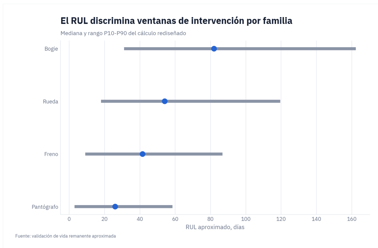
Figura. La mediana de vida remanente aproximada va de 26 días en pantógrafos a 82 días en bogies, con rangos P10-P90 también diferenciados. Fuente: validación de la vida remanente aproximada.
