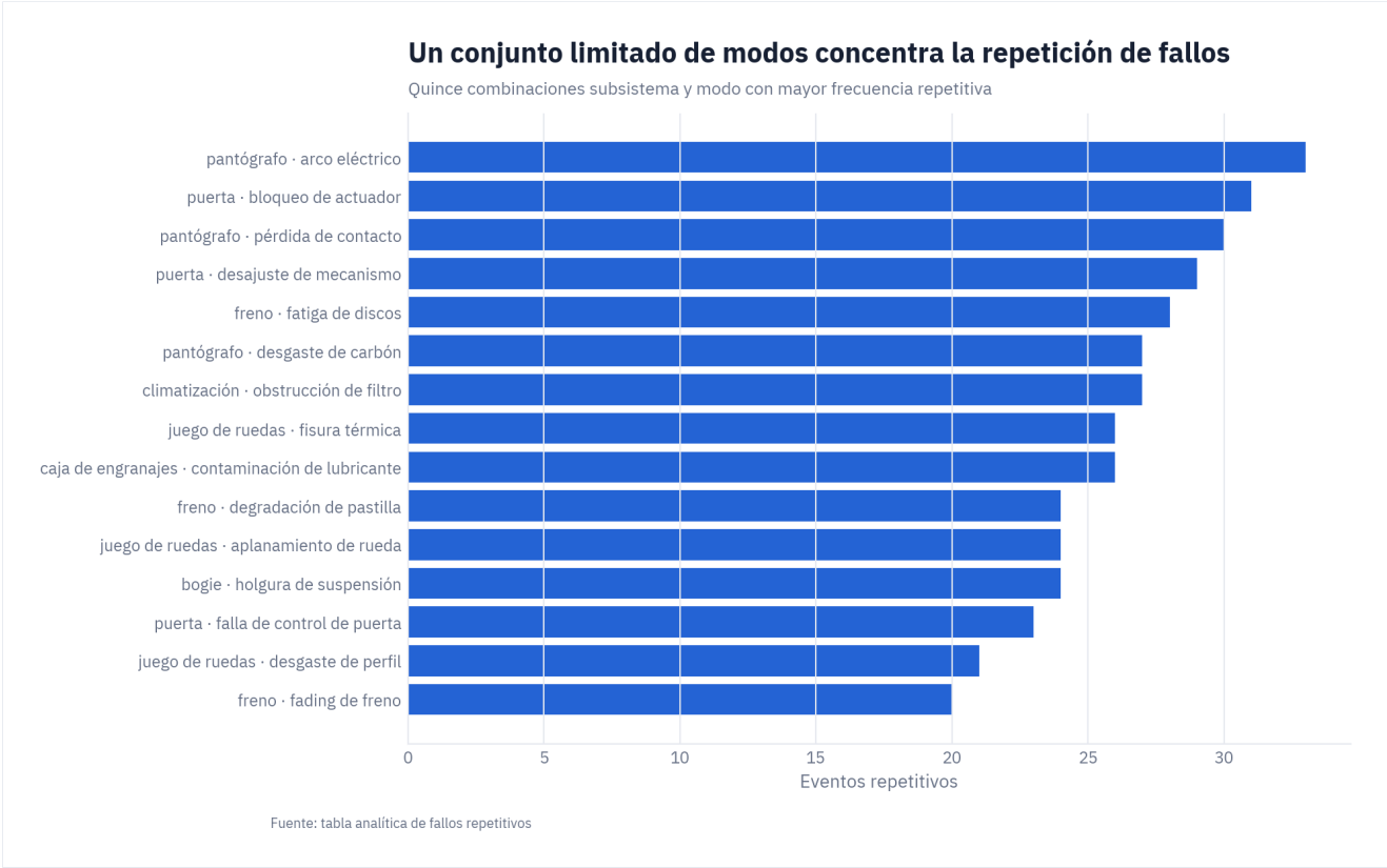
Figura. Los cinco modos con mayor repetición concentran el 28,4% de los eventos repetitivos incluidos en la clasificación. Fuente: tabla analítica de fallos repetitivos.
