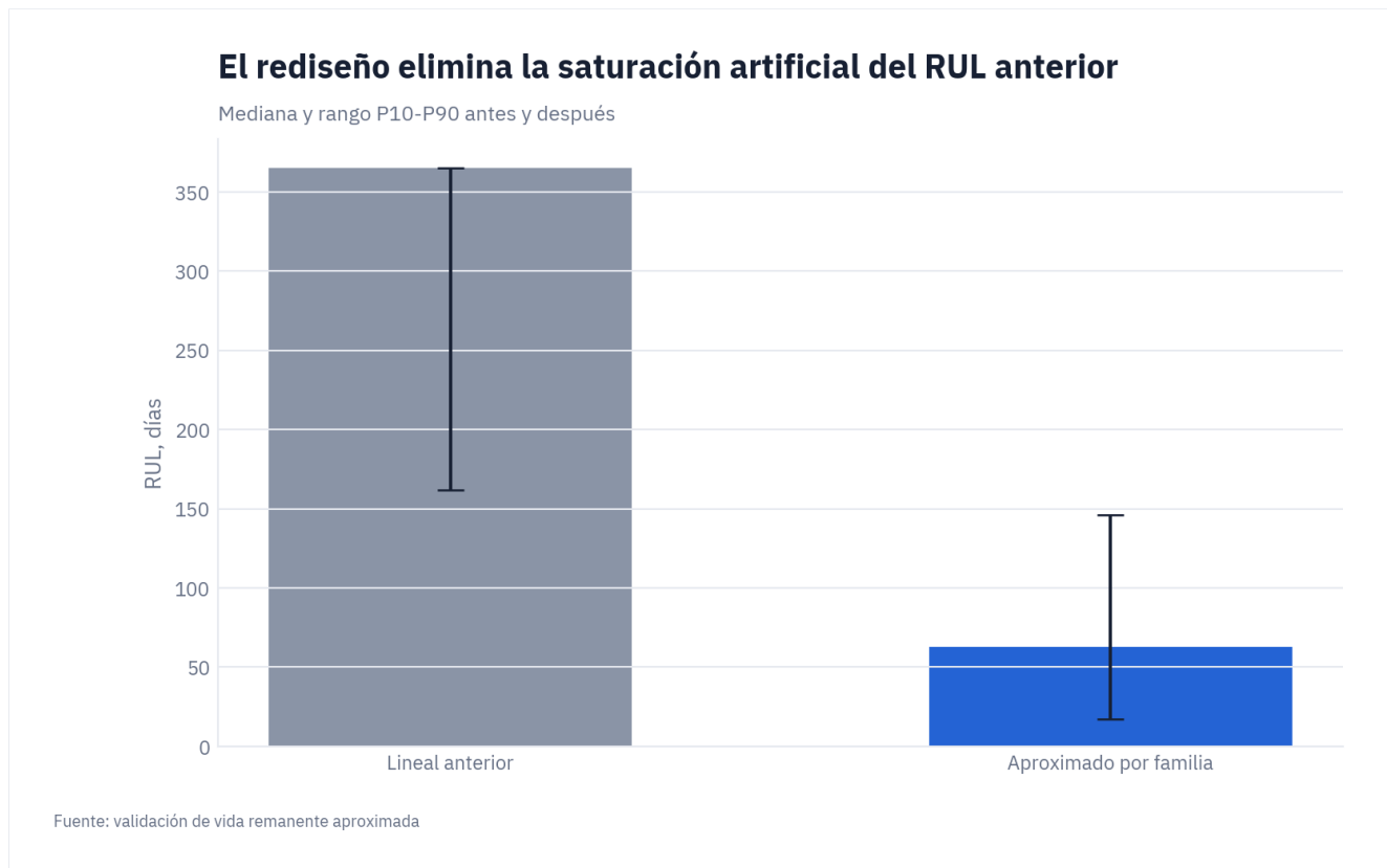
Figura. El modelo anterior concentraba el 72,3% de las observaciones en el tope de 365 días; el cálculo aproximado por familia reduce ese tope al 0,1%. Fuente: validación de la vida remanente aproximada.
