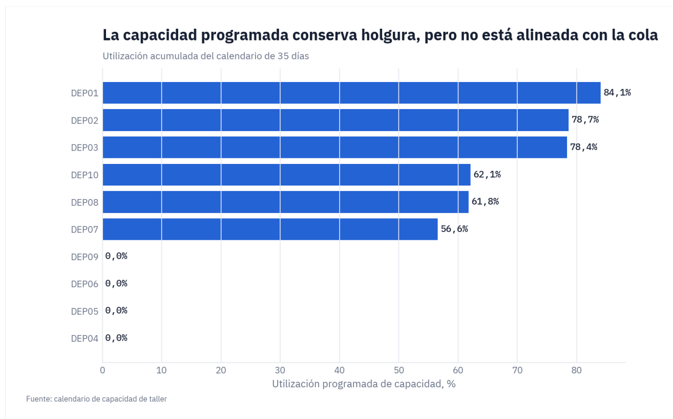
Figura. La utilización agregada del calendario de 35 días es 45,8%, lo que confirma que el bloqueo no se explica solo por falta absoluta de horas. Fuente: calendario de capacidad de taller.
