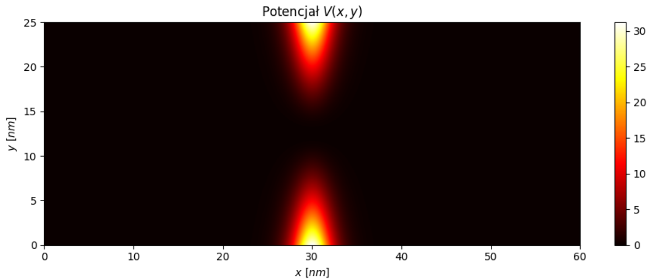
Rysunek 1: Mapa potencjału emulującego bramki
