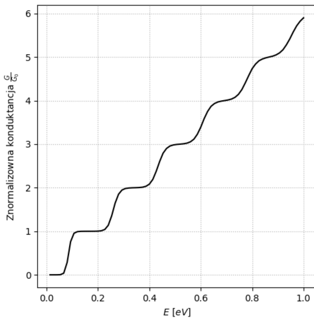
Rysunek 3: Wykres konduktancji od energii
