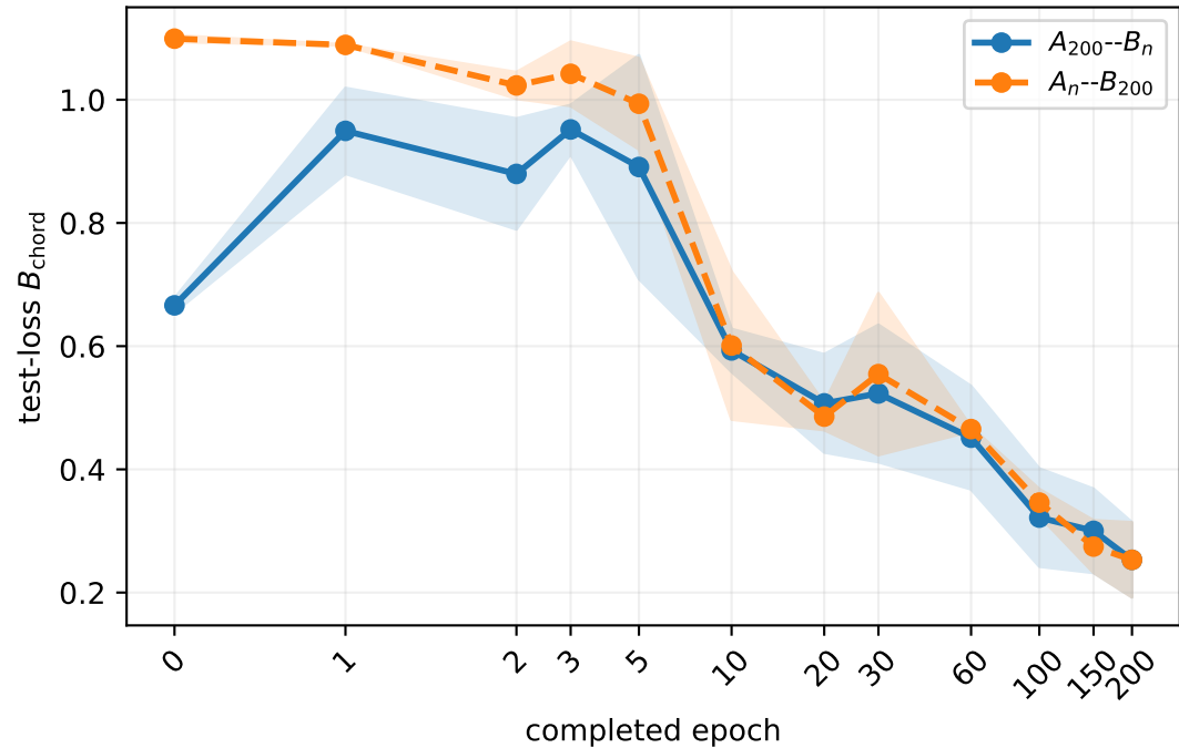
CIFAR-10 — VGG11
