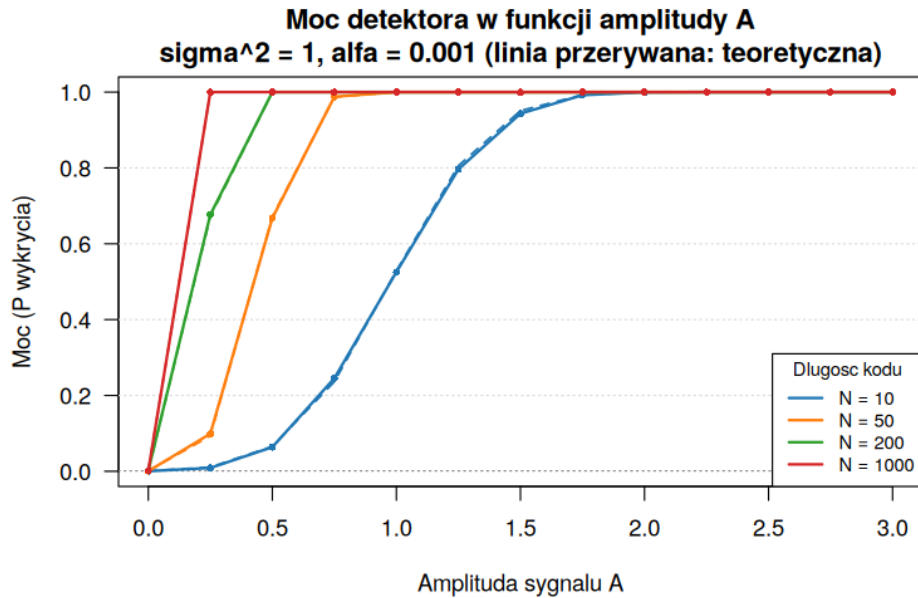
Rysunek 10: Empiryczna i teoretyczna moc detektora w funkcji amplitudy A dla różnych N ( \sigma^2 = 1 , \alpha = 0,001 ). Linie przerywane: wartości teoretyczne.
