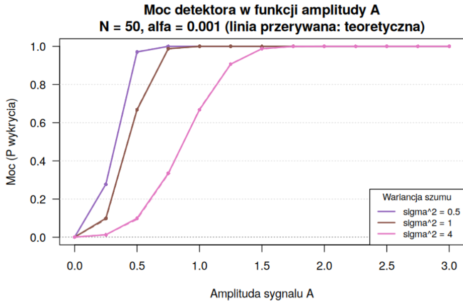
Rysunek 11: Empiryczna i teoretyczna moc detektora w funkcji amplitudy A dla różnych \sigma^2 ( N = 50 , \alpha = 0,001 ). Linie przerywane: wartości teoretyczne.
