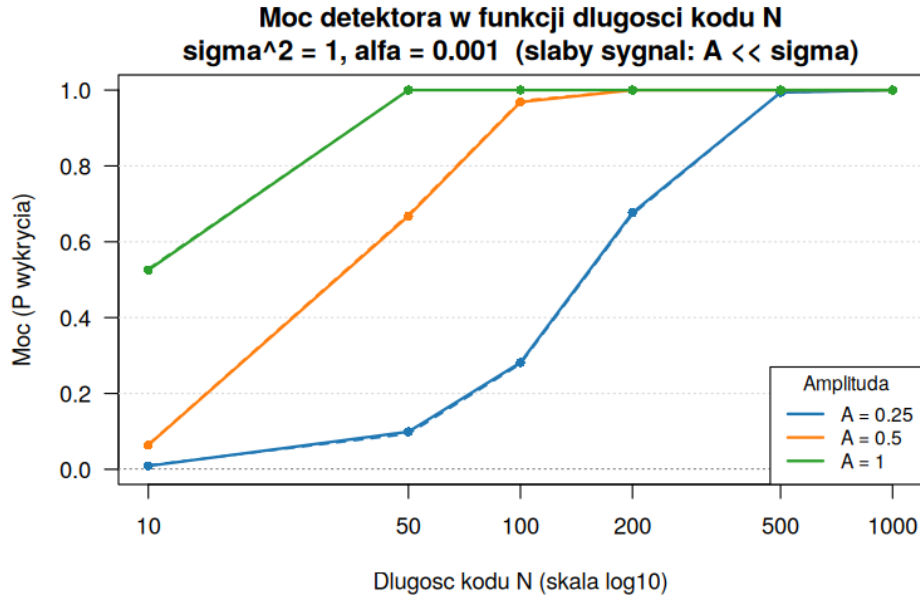
Rysunek 12: Moc detektora w funkcji długości kodu N dla słabych sygnałów ( \sigma^2 = 1 , \alpha = 0,001 ). Linie przerywane: wartości teoretyczne.
