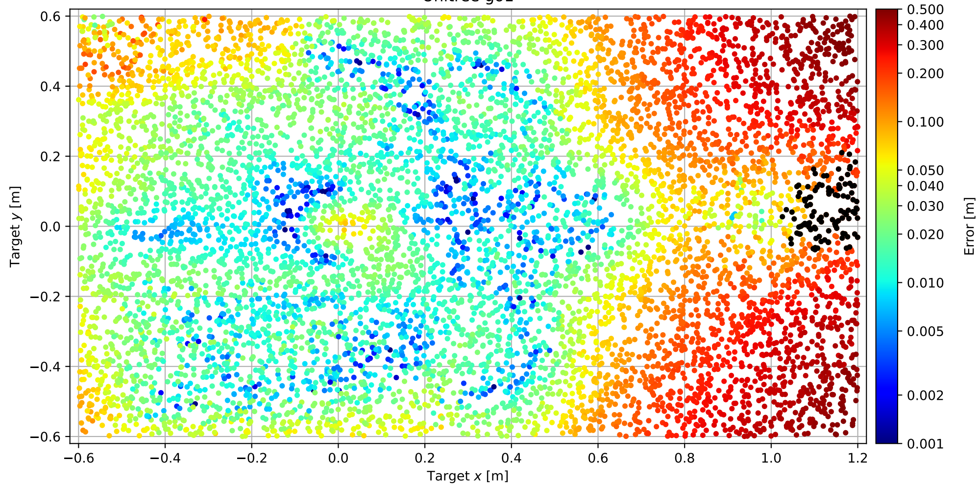
Unitree go1
