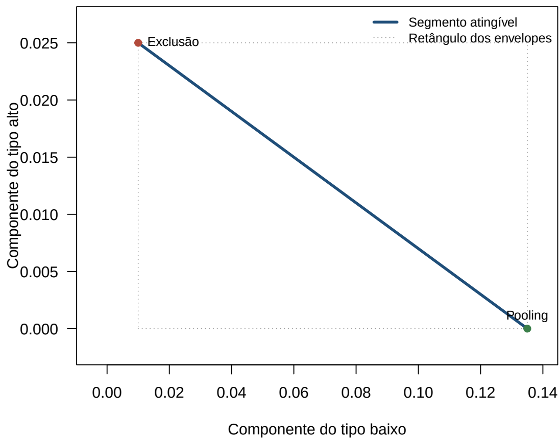
Figura 2: Segmento de payoffs com peso comum na fronteira o_1 = 1/m . Os limites de cada componente formam uma caixa, mas somente a linha corresponde a propostas do modelo.
