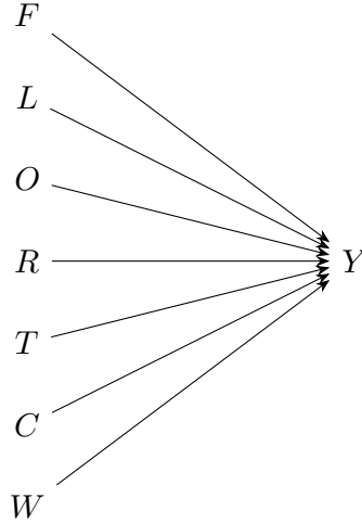
Figure 1: DAG do exemplo do incêndio. Função estrutural: Y = (F \wedge L \wedge O) \vee (R \wedge T) \vee (C \wedge W) . As variáveis binárias correspondem a fósforo aceso ( F ), folhas secas ( L ), oxigênio ( O ), raio ( R ), telhado inflamável ( T ), curto-circuito ( C ) e fiação inflamável ( W ).
