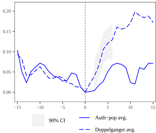
Trade/GDP (N=5)
