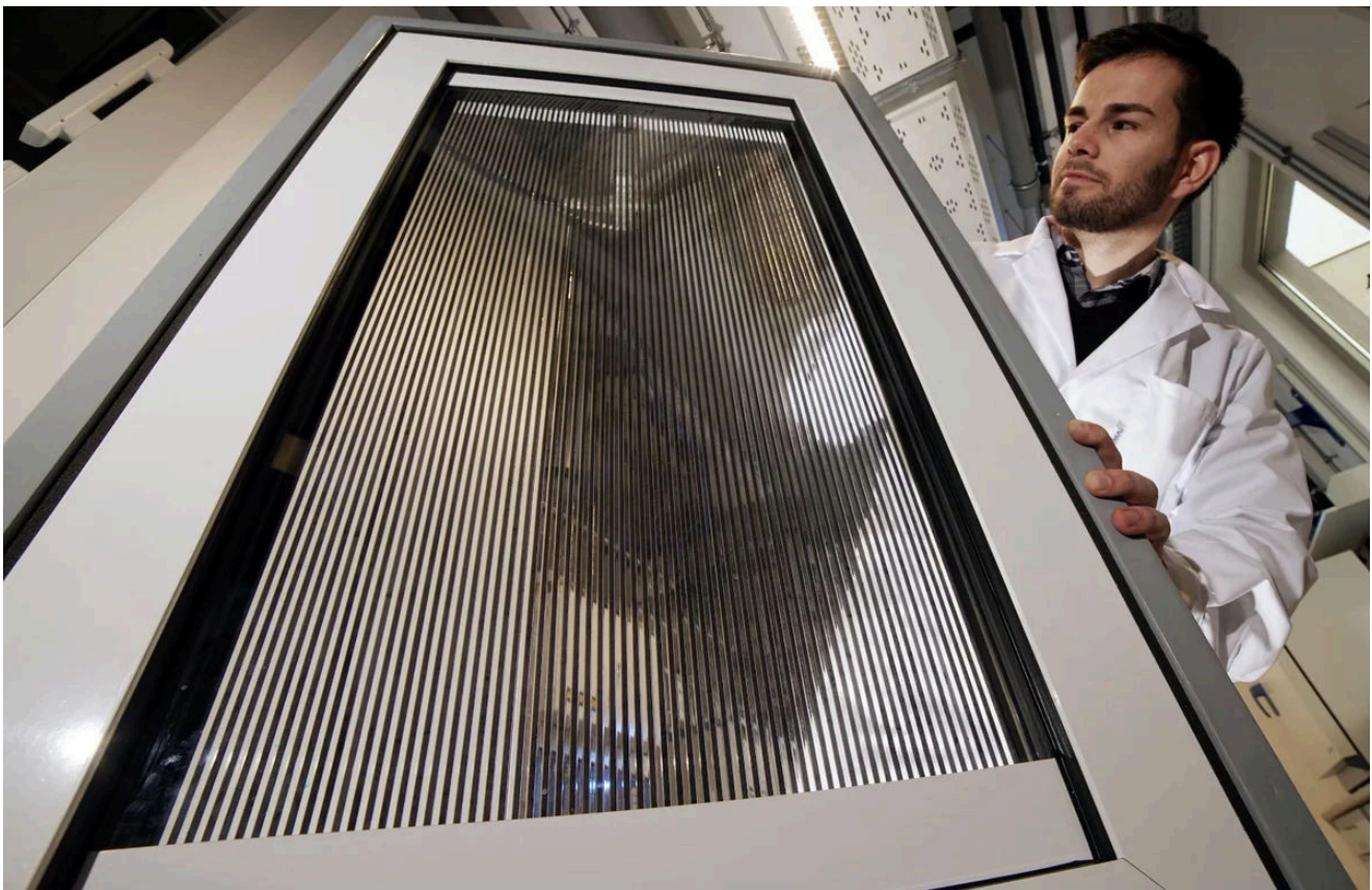
Abb. 2: LaWin-Prototyp mit magnetisch steuerbarer Fluidschicht — Eisen-Nanopartikel in der Kapillarstruktur regulieren Lichtdurchlässigkeit und Wärmeernste.
