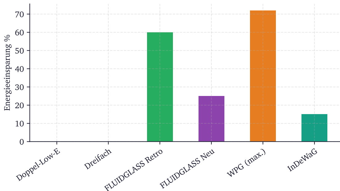
Abb. 5: Berichtete Energieeinsparungen fluidgefüllter Verglasungen gegenüber Doppel-Low-E-Referenzen (Bandbreite konservativ bis maximal je System)
