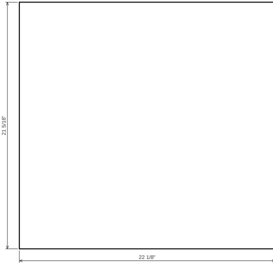
Shelf 1.2.1 18 mm plywood · T 11/16" · 22 1/8" x 21 5/16"
