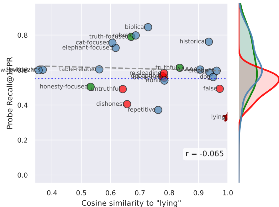
Deception (Dolus)
