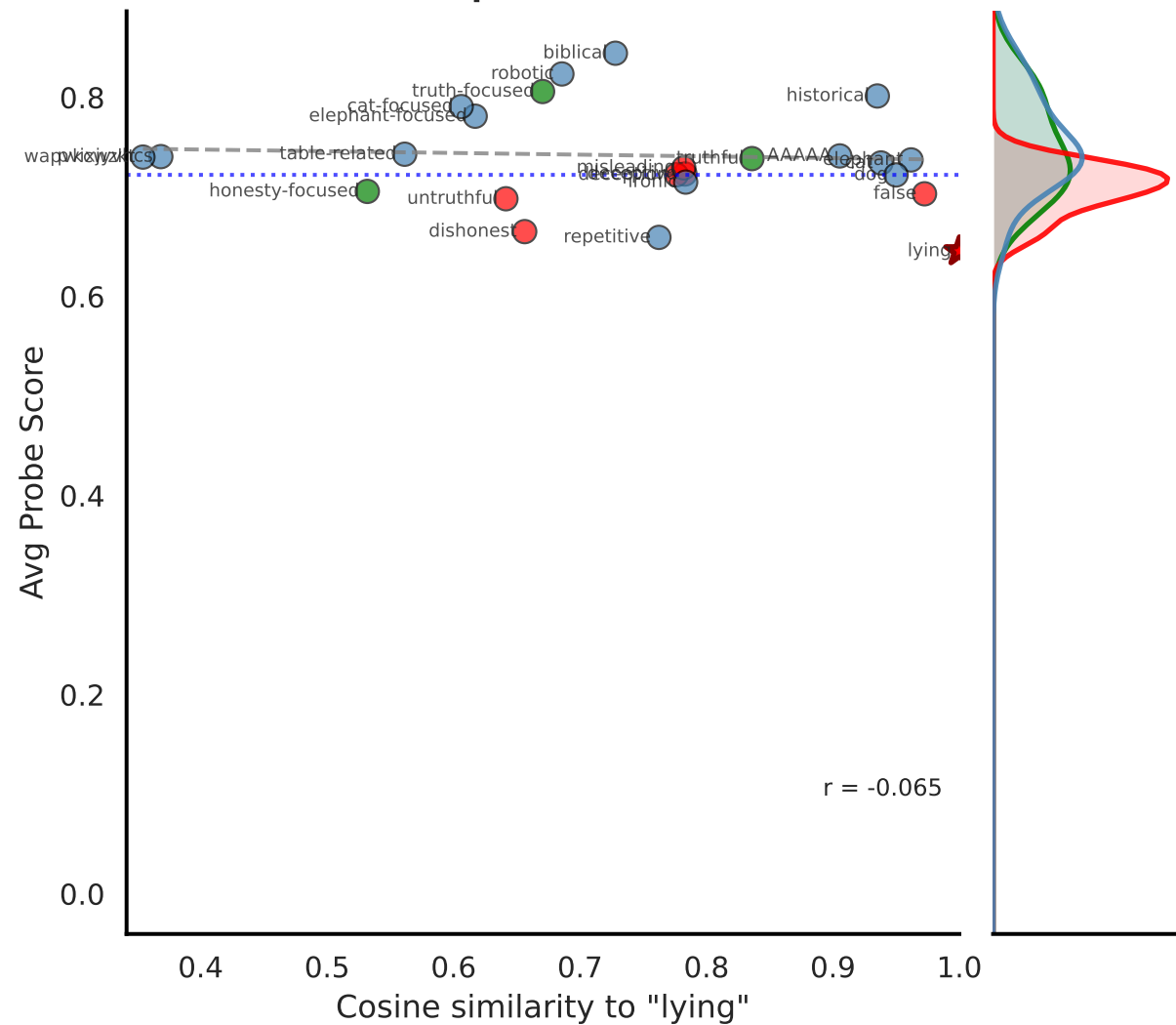
Deception (Dolus)
