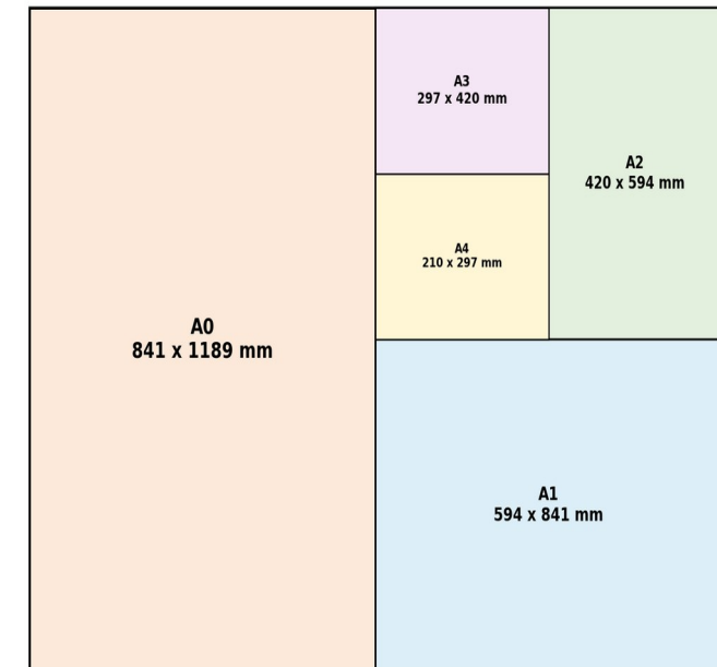
Fig. 2.1 — Anidamiento de la serie A, del A0 al A4.
