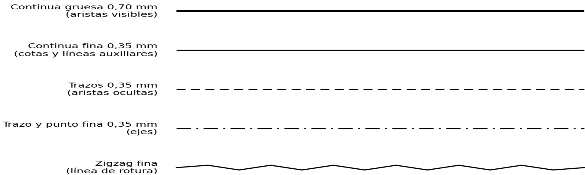
Fig. 2.2 — Continua gruesa: aristas visibles · Continua fina: cotas y auxiliares · Trazos: aristas ocultas · Trazo y punto: ejes · Zigzag: roturas. Trazo y punto con extremos gruesos: trazos de planos de corte.
